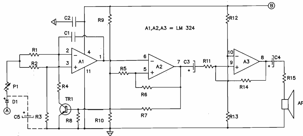
figura 2 Il voltmetro.
