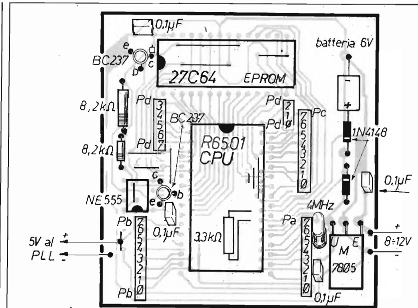
figura 10 Piano di montaggio della scheda CPU.
