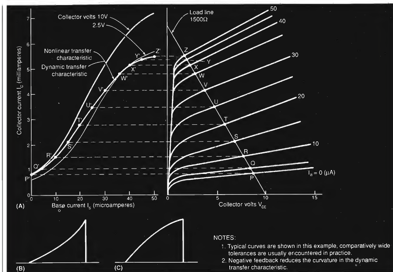
figura 6 Rappresentazione grafica del processo di predistorsione: (A) caratteristica di trasferimento dinamica di un transistor bipolare; (B) predistorsione a bassa polarizzazione; (C) predistorsione ad alta polarizzazione. Per completare il processo di linearizzazione si fa uso della reazione negativa.
