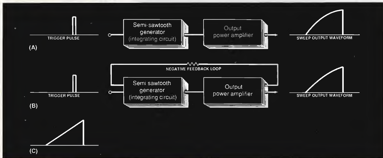
figura 5 Circuiti formatori d'onda nello sweep verticale di un ricevitore TV: (A) configurazione fondamentale; (B) un dente di sega parzialmente linearizzato per controreazione; (C) un dente di sega ideale, che si otterrebbe per effetto di un tasso di controreazione infinito.
