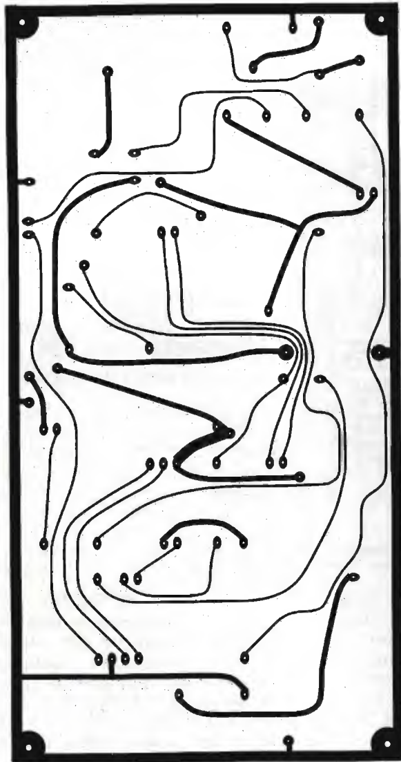
figura 6c Modulo sintesi/microprocessore, circuit stampato, lato componenti.
