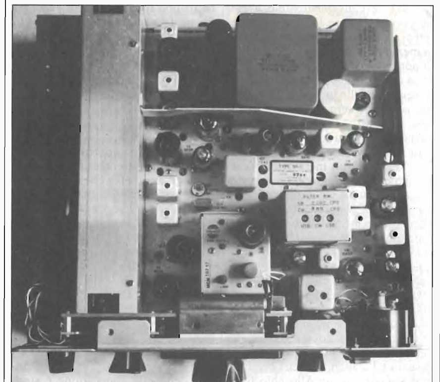
foto 3 Vista interna: a sinistra il lungo rettangolo contiene il meccanismo del VFO. A destra si può notare la scatola con i filtri.
