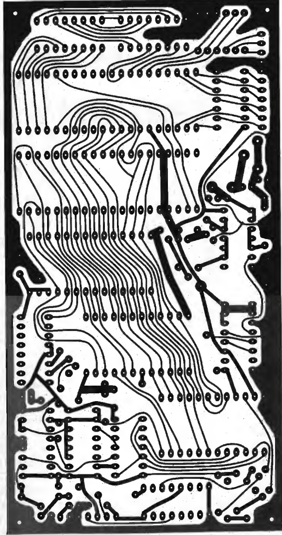
figura 6d Modulo sintesi/microprocessore, circuit stampato, lato saldature.
