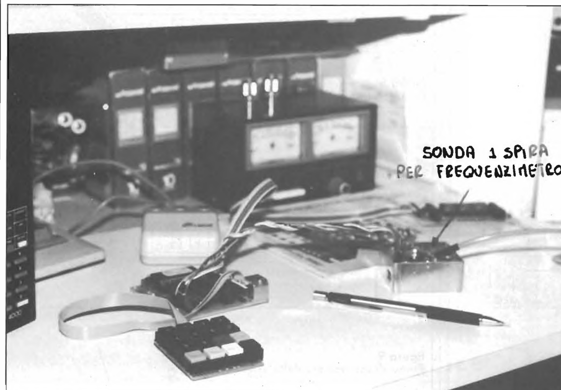
foto 4 Altre prove del generatore: una semplice sonda-spira serve per l'accoppiamento col frequenziometro, mentre un ricevitore, a destra, consente di verificare la presenza di spire.
