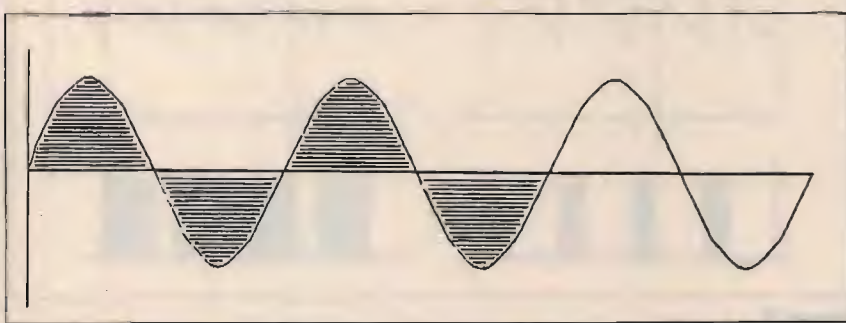
figura 6 "In un sistema proporzionale migliorato, vengono lasciati transitare cicli interi. In questo modo, la potenza viene regolata modificando il rapporto tra cicli inviati al carico (indicati col tratteggio) e cicli bloccati".
