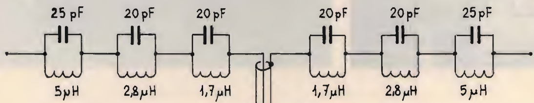
schema elettrico
