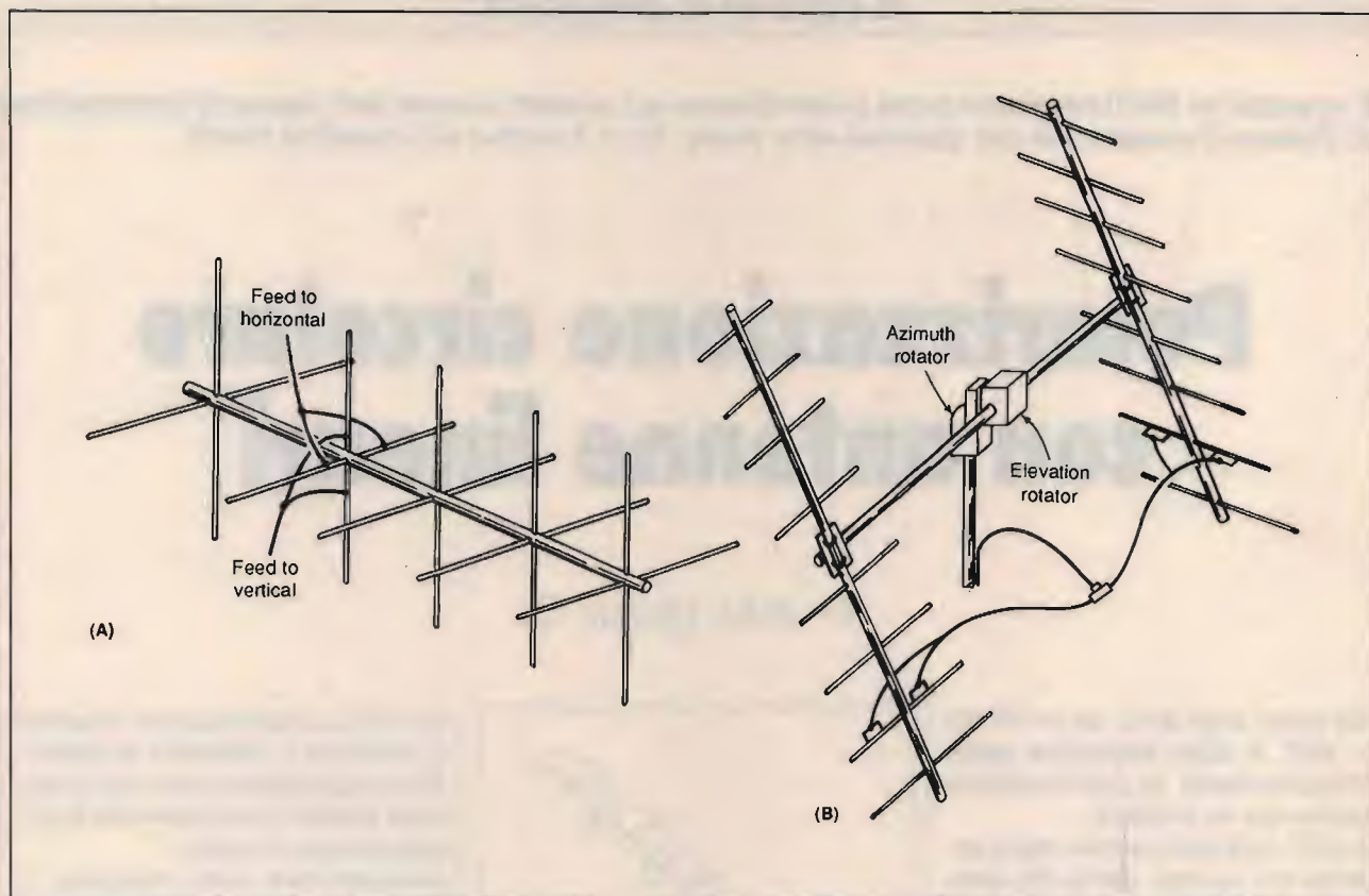
figura 2 "In A, una Yagi incrociata con entrambe le antenna montate sullo stesso boom. In B, un'altra versione di Yagi incrociata, con ciascuna antenna montata su un boom indipendente. In entrambi i casi, i piani delle due antenne sono reciprocamente perpendicolari".
