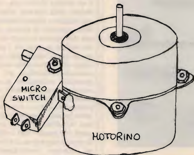
figura 1 Il trapanino come si presenta con l'interruttore montato.
