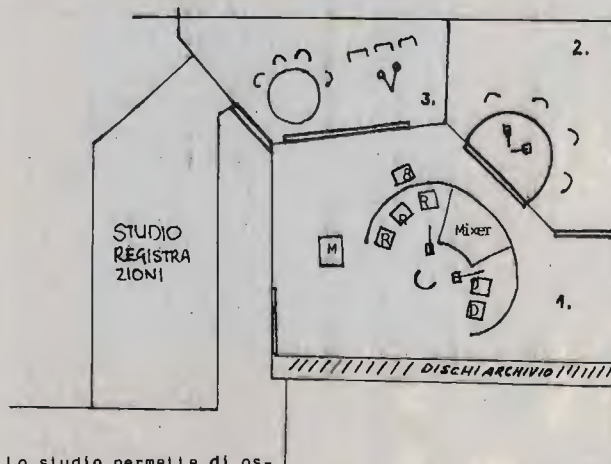
SCHEMA DI MASSIMA DELLO STUDIO DI RADIOCADENA TALAVERA
