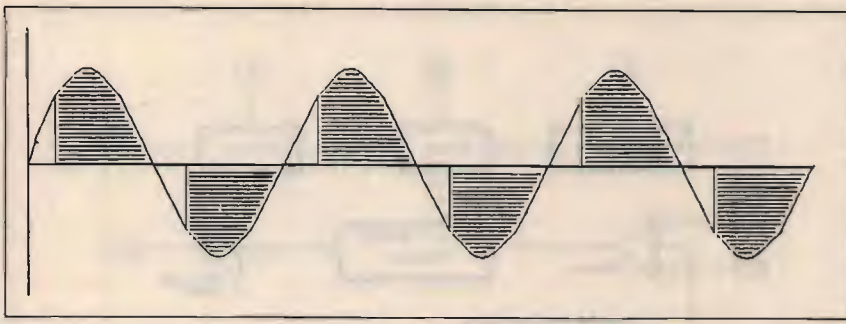
figura 5 "L'aggiunta del controllo di fase consente ad un sistema proporzionale di tipo convenzionale di comportarsi come un variatore di luminosità per lampade, campionando la sinusoide della corrente di rete per regolare la potenza".
