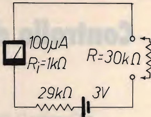
figura 2 Schema pratico di ohmetro. Se la resistenza in prova è da 30 \text{ k}\Omega , l'indice si fermerà a metà scala, perché anche la resistenza interna dell'ohmetro è 30 \text{ k}\Omega . L'amperometro segnerà 50 \mu\text{A} .
