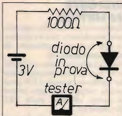
figura 7 Controllo di un diodo se l'ohmetro è in panne. Si possono distinguere i diodi al germanio da quelli al silicio per la diversa soglia di conduzione e per la diversa corrente inversa.
