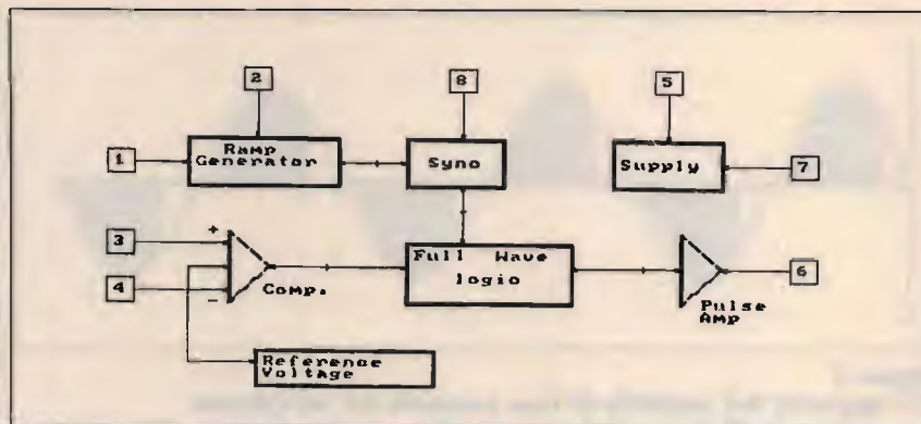
figura 7 "L'integrato Telefunken U217B svolge diverse funzioni, che normalmente richiederebbero l'impiego di numerosi integrati ed altri componenti".
