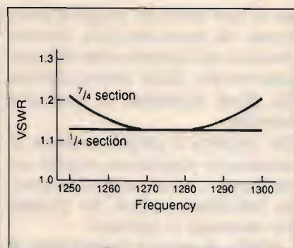
figura 4 "Una comparazione del ROS nell'arco della intera gamma operativa impiegando una sezione di adattamento da 1/4 e da 7/4 di lunghezza d'onda".
