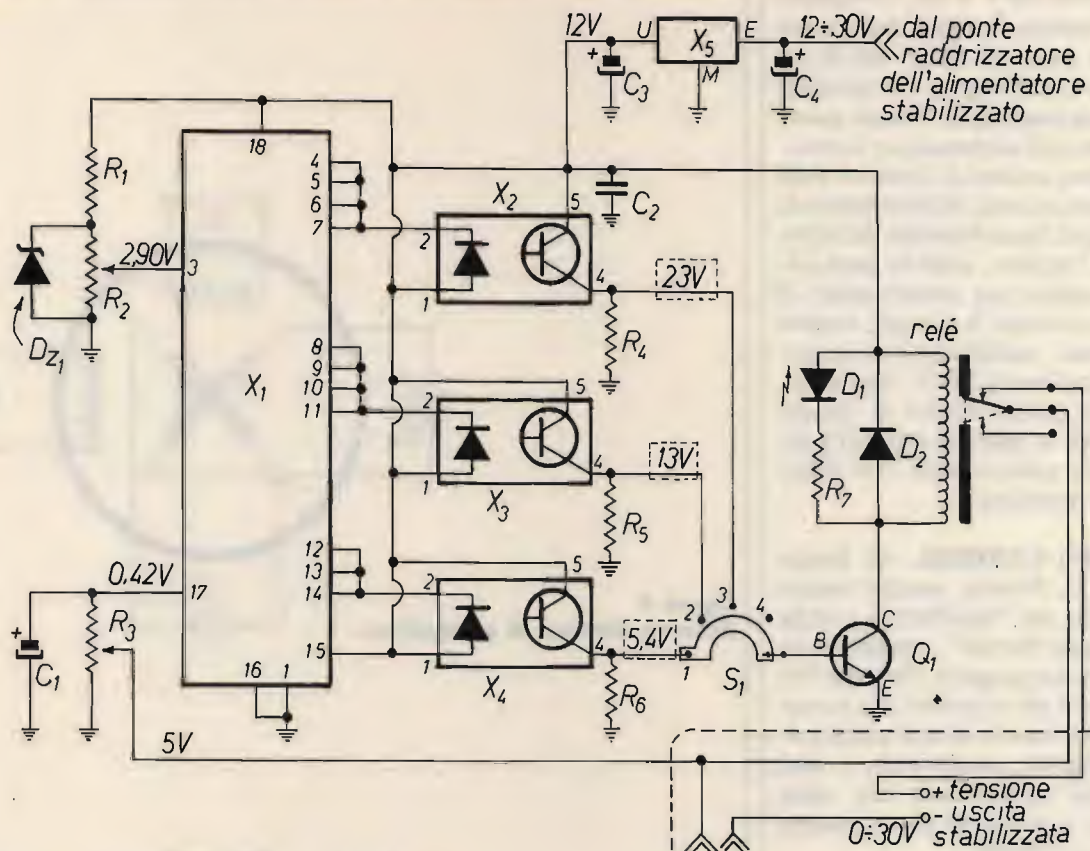
figura 3 Protezione in tensione su un alimentatore variabile.
