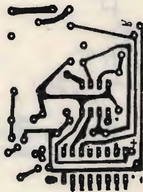
figura 6 Circuito stampato del timer, lato rame.
