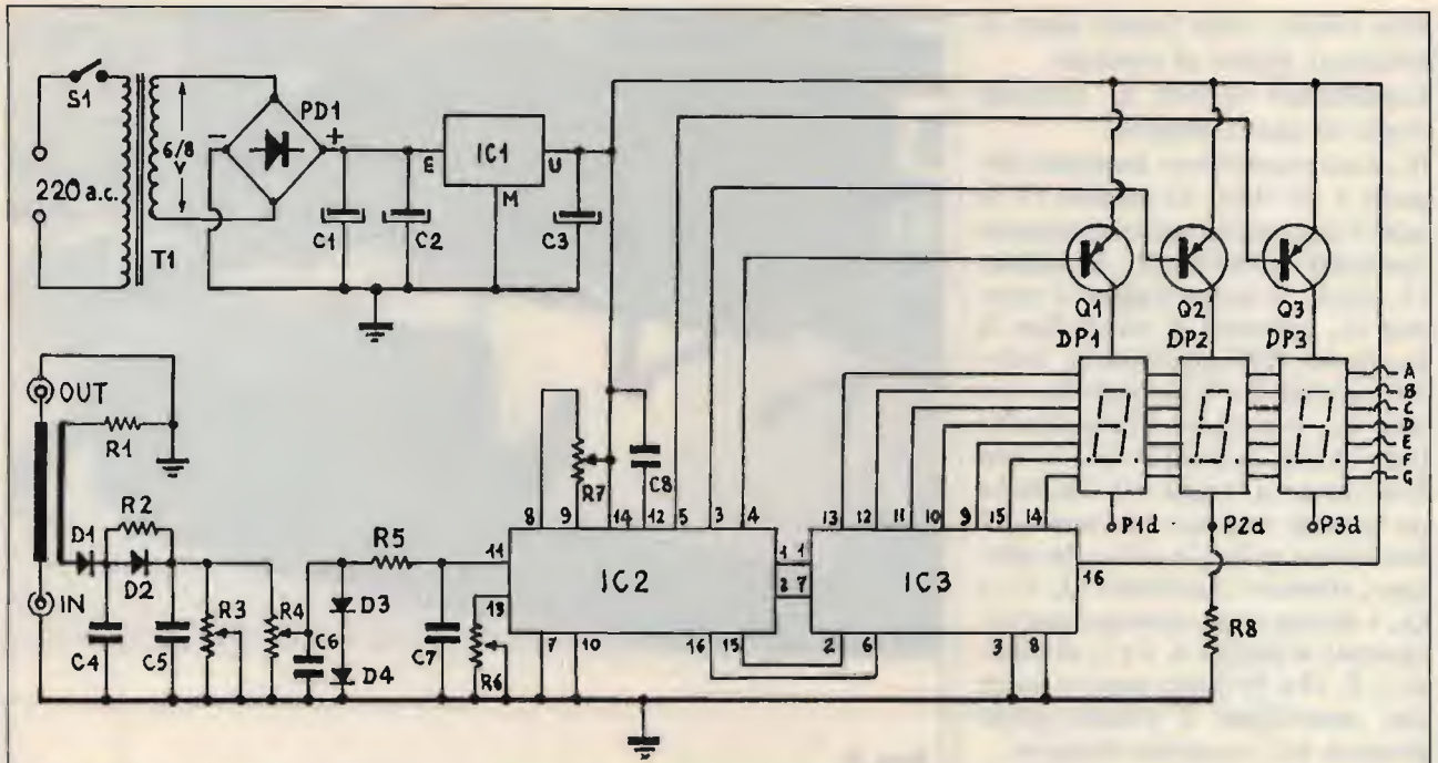
figura 8 Schema elettrico.
