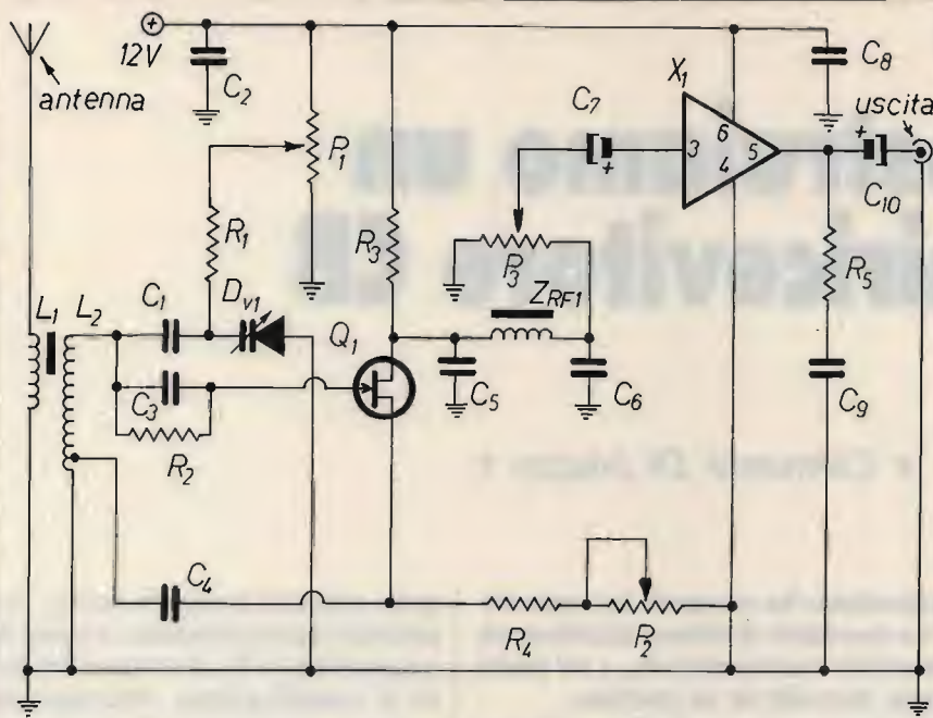
figura 1 Schema elettrico e componenti.
