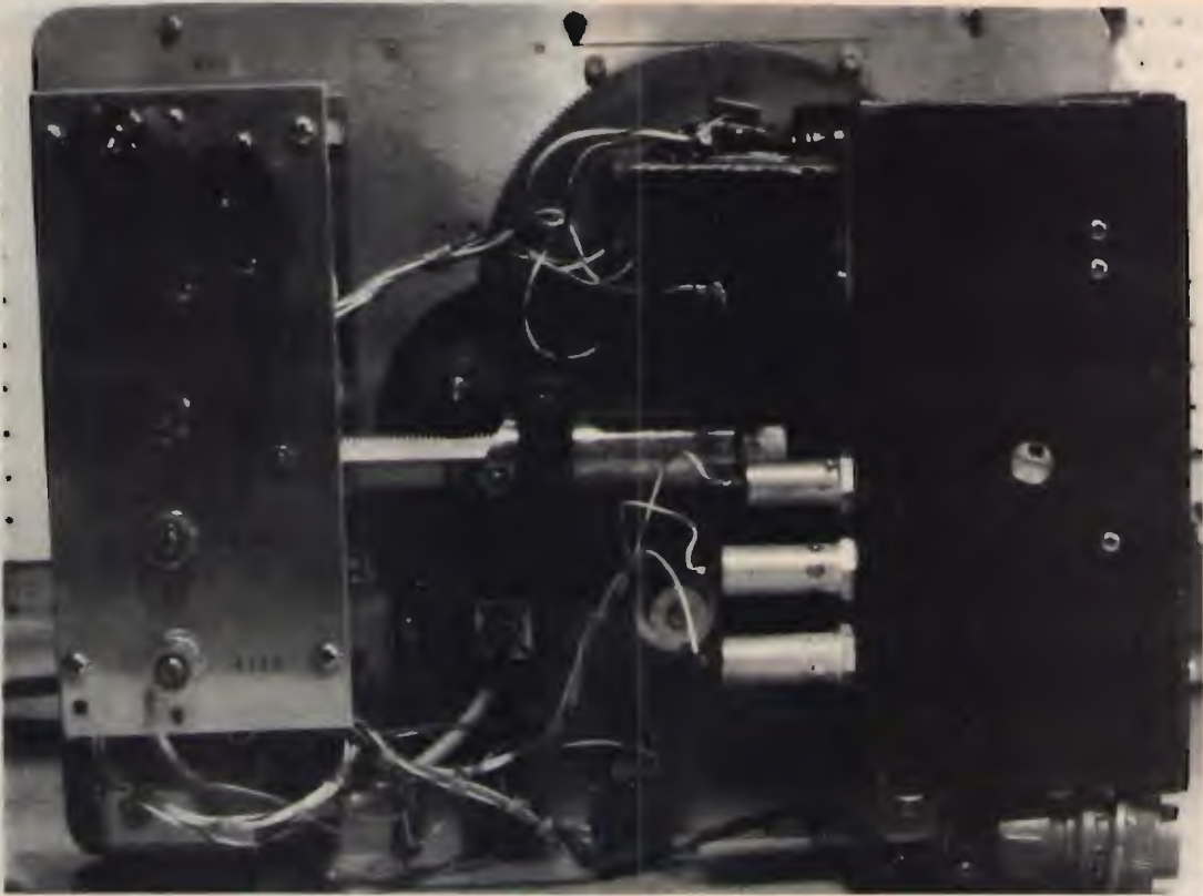
foto 3 Vista interna. Al centro è ben visibile il pistone per il prelievo attenuato della RF in uscita.
