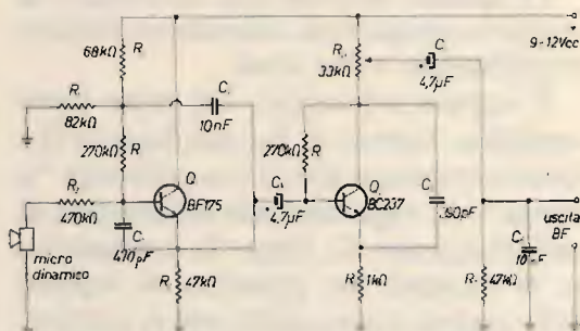
Schema elettrico completo del preamplificatore microfonico per RTX.
