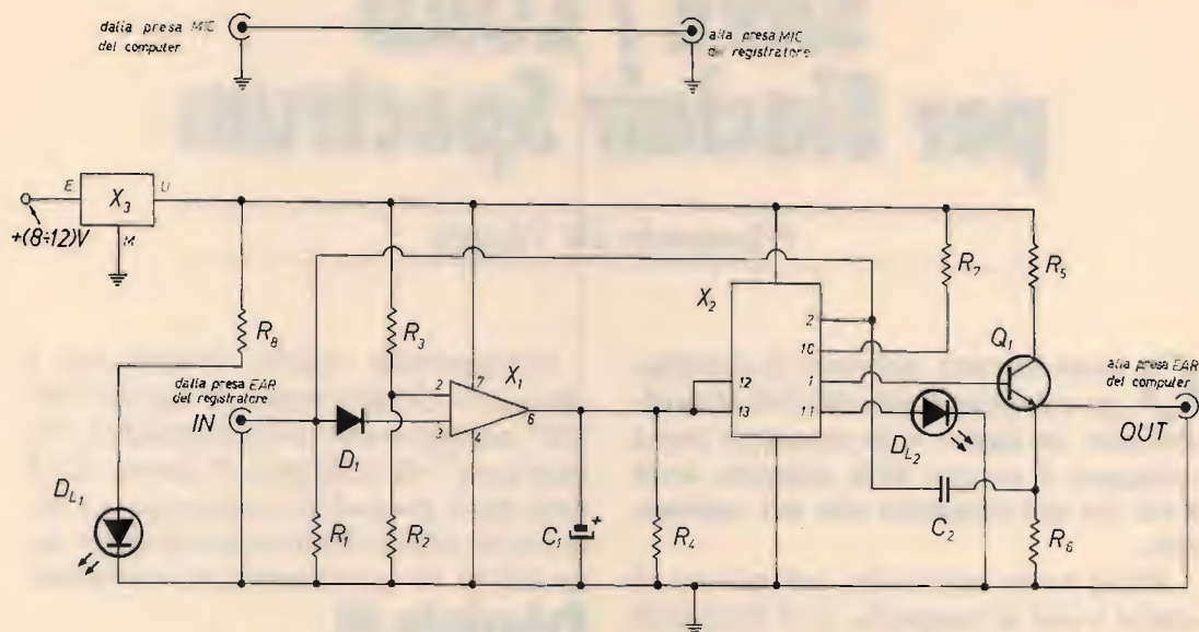
figura 2 Schema elettrico.
