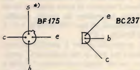
CONNESSIONI DEI TRANSISTORI IMPIEGATI (VISTI DA SOTTO).
