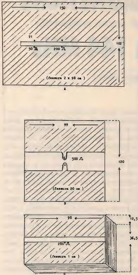
figura 1 Dimensioni e forme dei dipoli descritti nel testo (misure espresse in centimetri):
