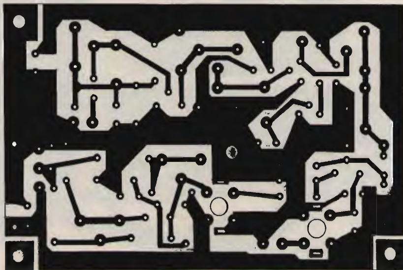
CIRCUITO STAMPATO (1:1)
