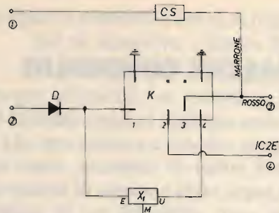
Schema elettrico
