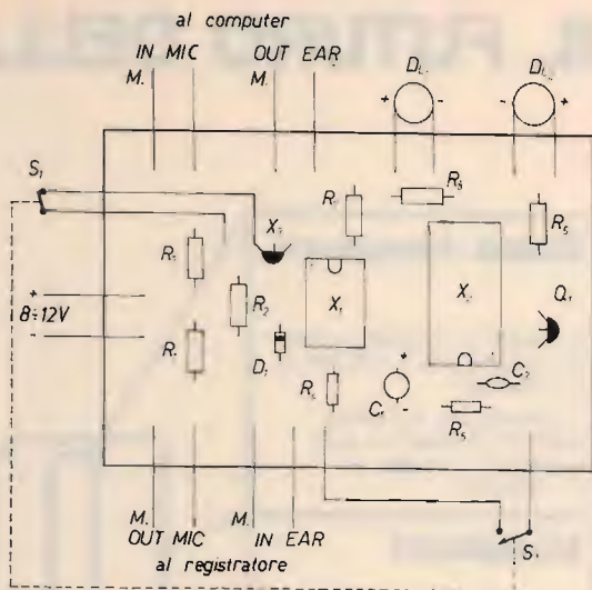
figura 5 Lato componenti; schema pratico di montaggio.
