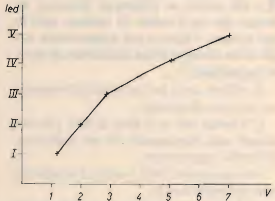
Approssimazione con 5 led di una funzione logaritmica.
