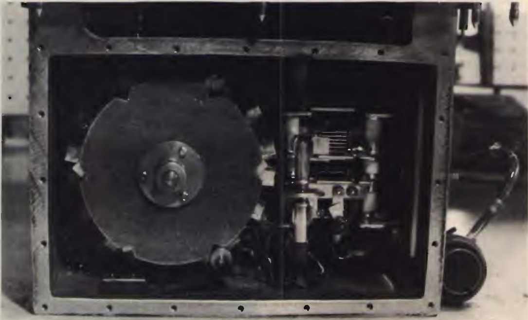
foto 4 Interno del VFO: visibile il retro del tamburo portabobine e la microscopica valvola oscillatrice.
