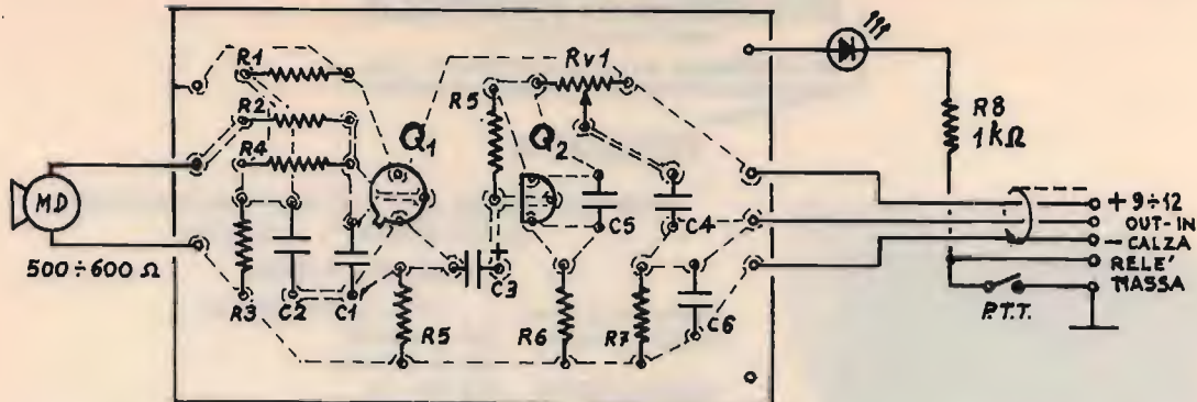
Schema pratico di montaggio del preamplificatore per RTX, lato componenti.
