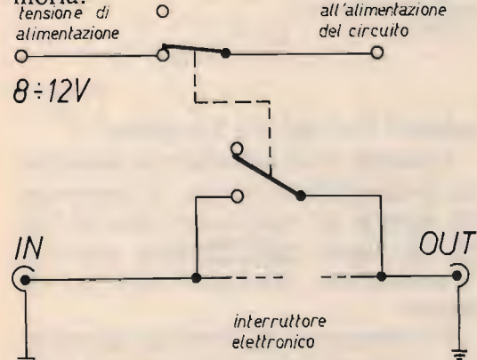
figura 1 Schema del commutatore.
