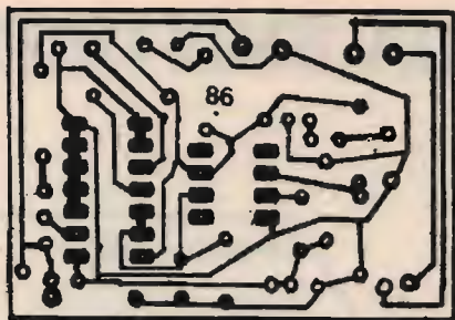
figura 4 Dimensioni della basetta in scala 1:1, lato rame.
