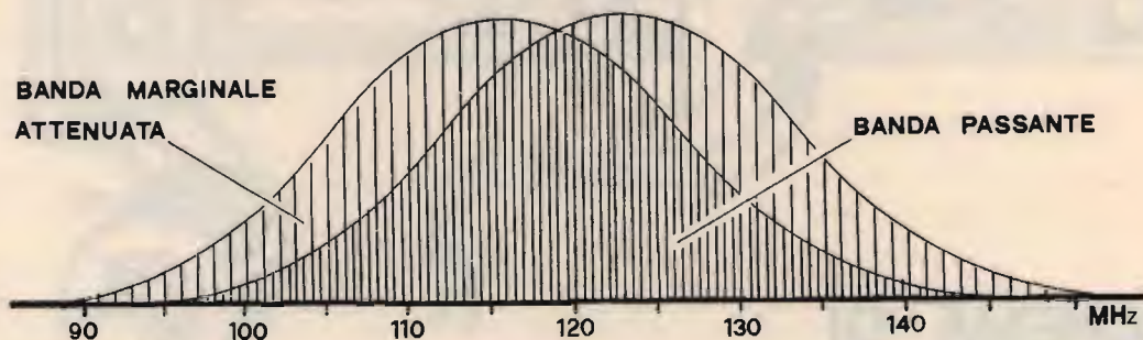
BANDA PASSANTE DEL PREAMPLIFICATORE-PRESELETTORE ( Q_1, Q_2 E ANNESSI)
