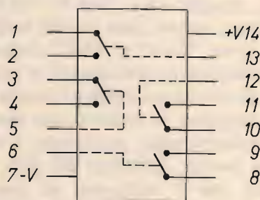
figura 3 Configurazione dei piedini dell'integrato X 2 (CD4066).
