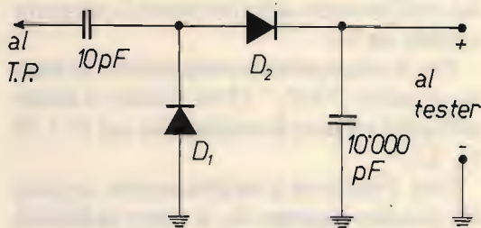
D_1, D_2 diodi al Germanio.
