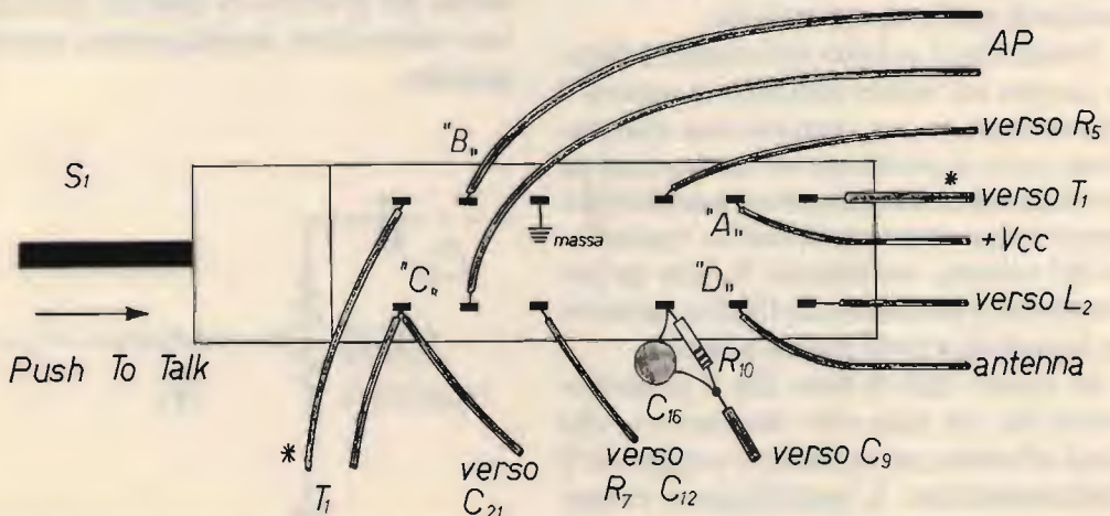
Particolare dei collegamenti al deviatore S 1 . Restano uguali anche per un deviatore a slitta.
