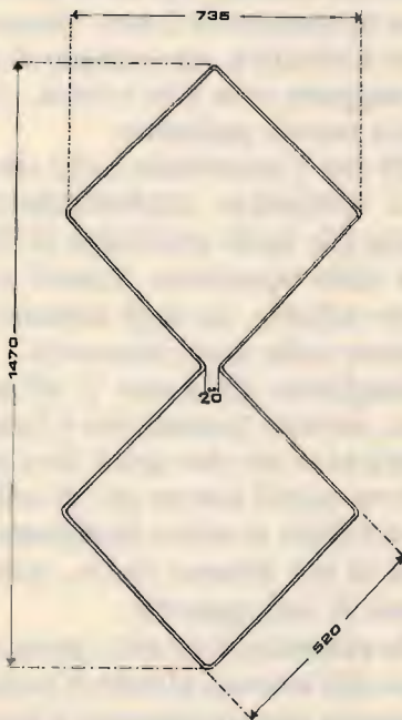
DETTAGLIO DELL'ELEMENTO RADIANTE
