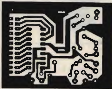
CIRCUITO STAMPATO CODER (1:1)
