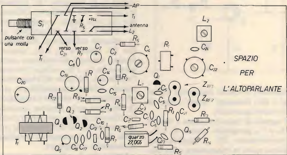
Disposizione dei componenti; non compaiono C 16 e R 10 che sono sistemati in "aria" (vedi foto). Le dimensioni reali sono di 85 x 42 mm.
