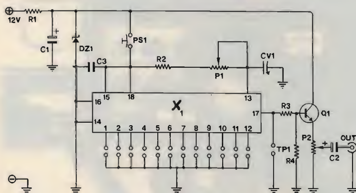
SCHEMA ELETTRICO DEL CODER
