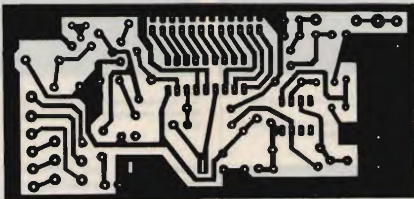
CIRCUITO STAMPATO DEL DECODER
