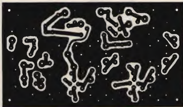
figura 2 Circuito stampato a faccia singola, lato rame.
