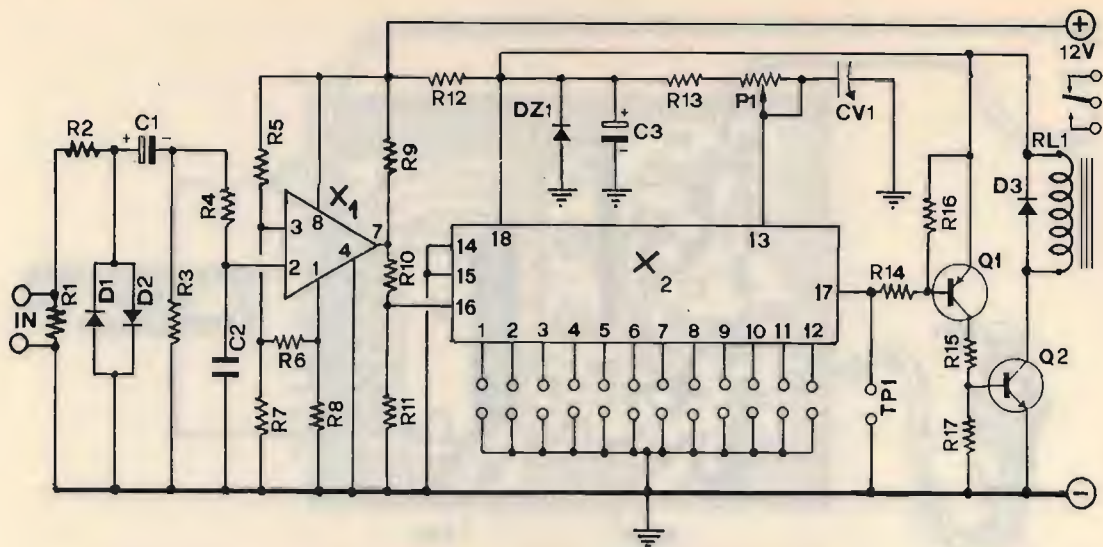
SCHEMA ELETTRICO DEL DECODER
