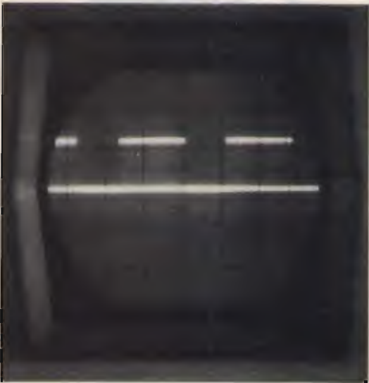
foto 7B Forma d'onda dei segnali prelevata sul piedino 7 di X_1 : la ricostruzione del segnale originale è presso che perfetta.
