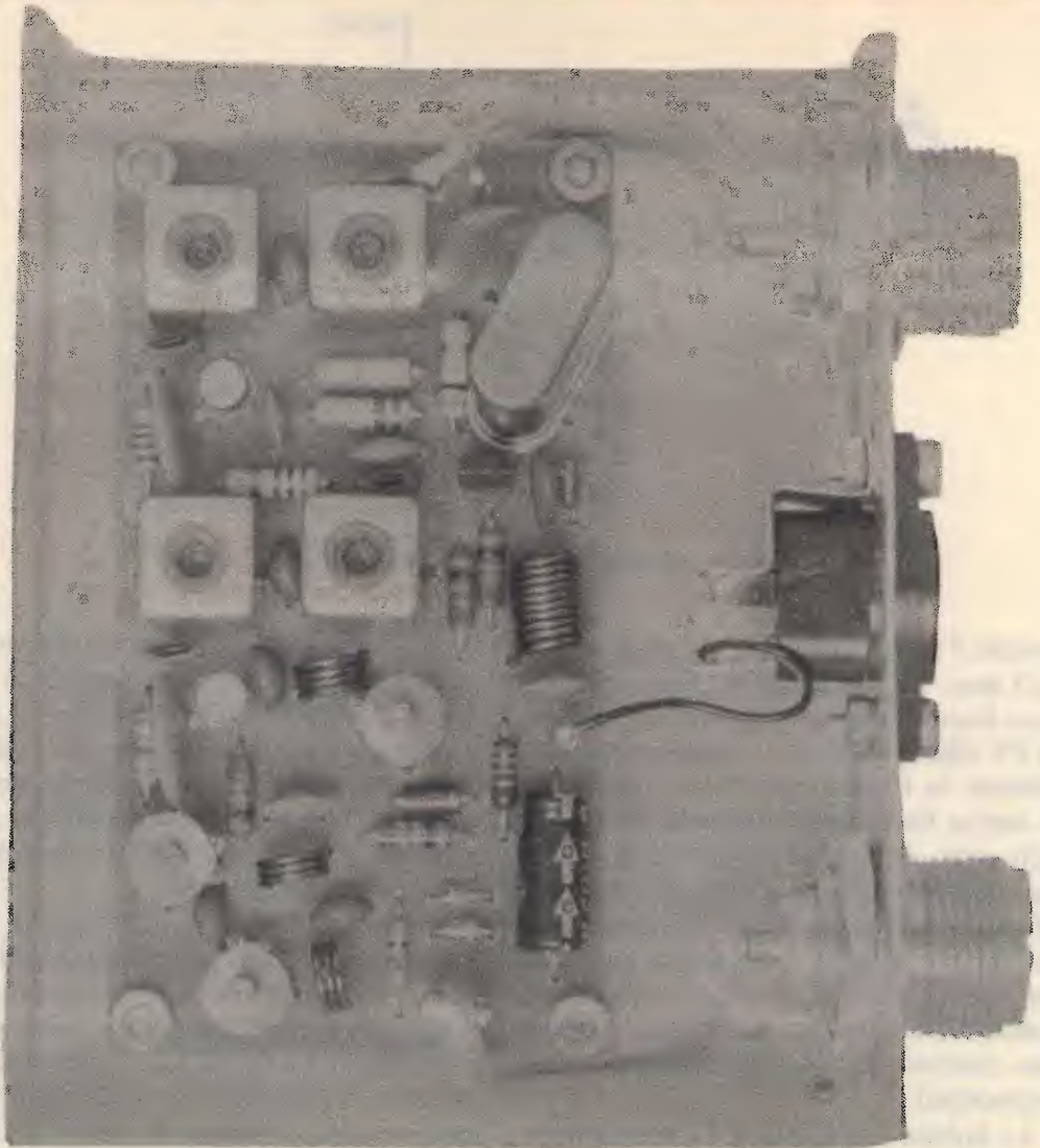
Upconverter, versione 28→144 MHz.
