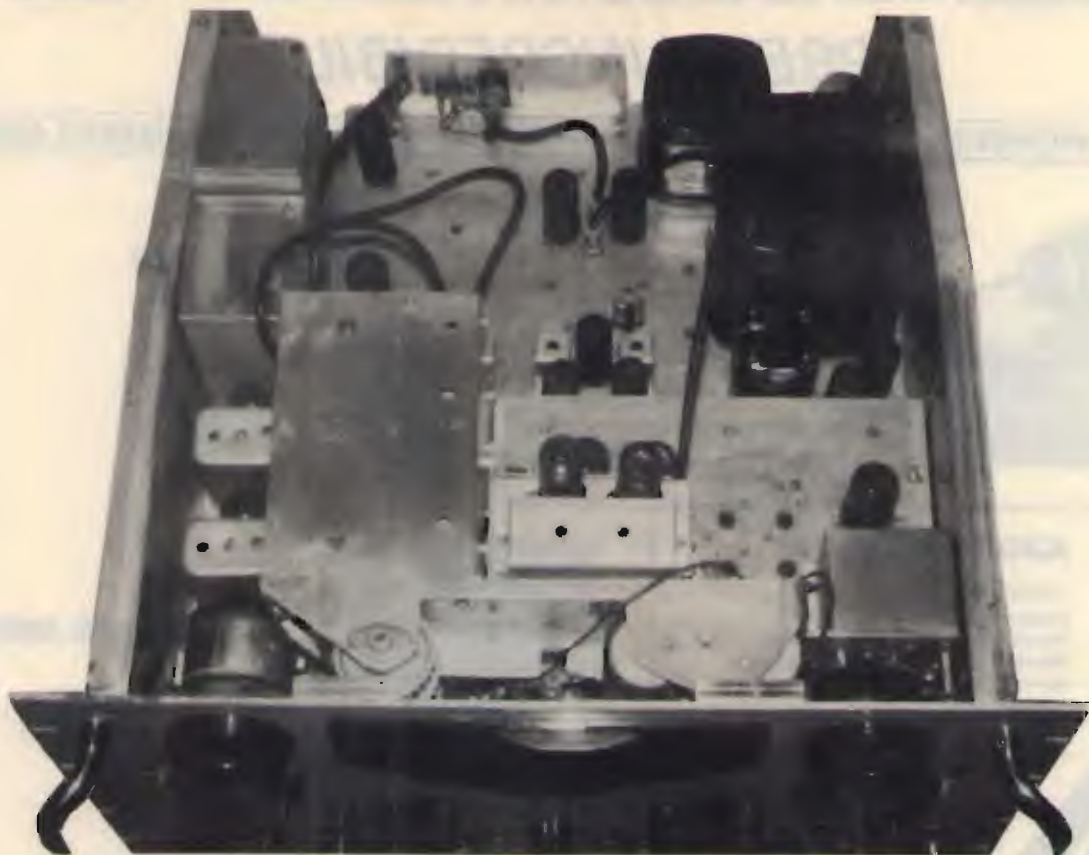
Vista interna, superiore, del RA-17. Notare il meccanismo per la scala a film, e il piccolo altoparlante di servizio.
