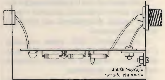
figura 9 Sezione trasversale.
