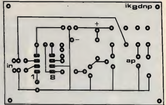
CIRCUITO STAMPATO (lato rame)
