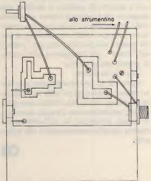
figura 10 Vistu dall'alto.
