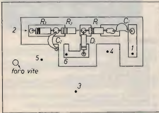
figura 7 Da collegare con ponticelli i numeri uguali sulle due facce
