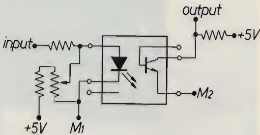
4) proporzionale in controfase
