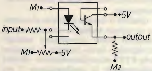
4) proporzionale in controfase
