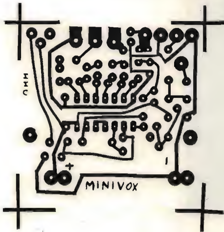
figura 2 Circuito stampato.
