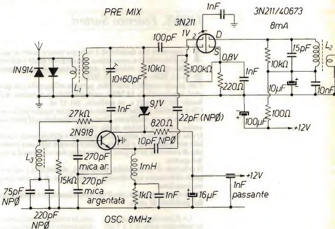
figura 1 Schema elettrico del convertitore 7 → 14 MHz
