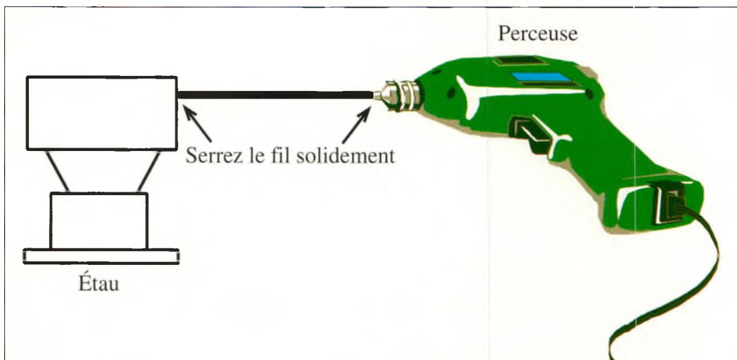
Fig. 1- Une méthode simple et rapide pour raidir un fil de cuivre épais ou un tube de cuivre de faible diamètre. Assurez-vous de bien serrer le fil à chaque extrémité et de porter des lunettes de protection.
