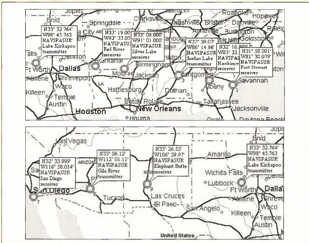
Les sites des stations NAVSPUR. Ces radars sont audibles vers 210 MHz lorsque leur rayon croise la lune.
