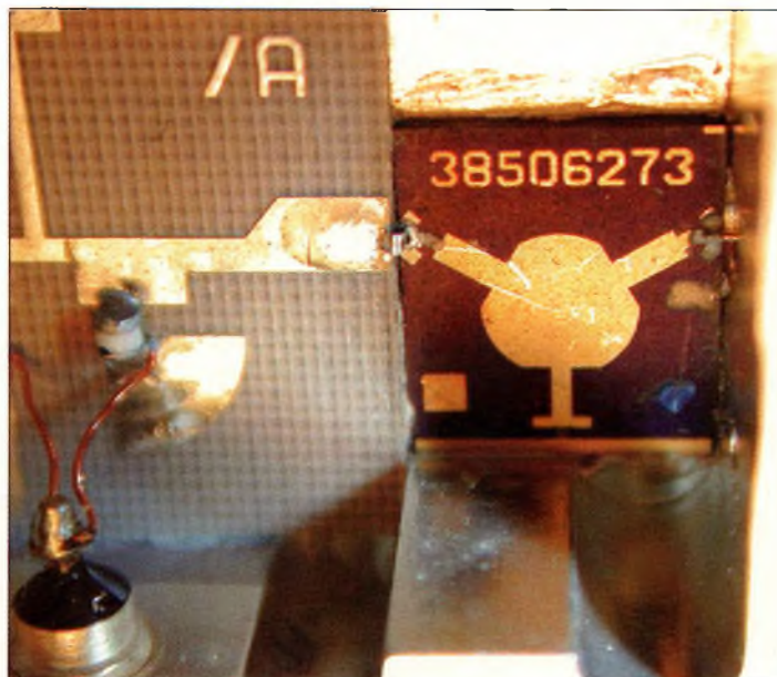
L'intérieur d'un isolateur.
