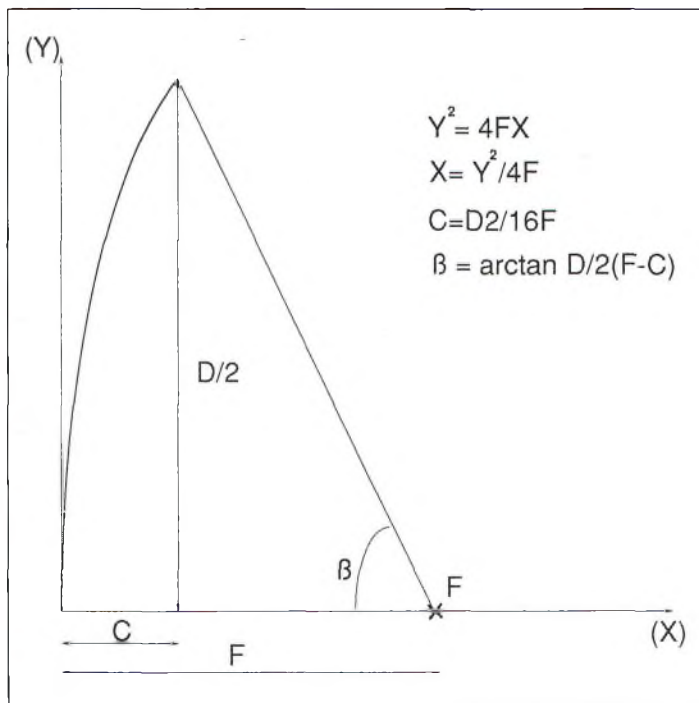
Fig. 2 et 2a — Calcul de la parabole primifocus.
