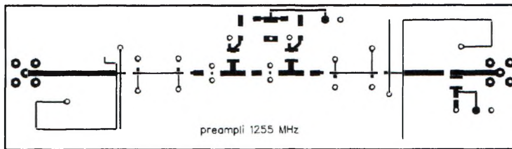
Fig. 4 — Le circuit imprimé du préamplificateur 1255 MHz.
