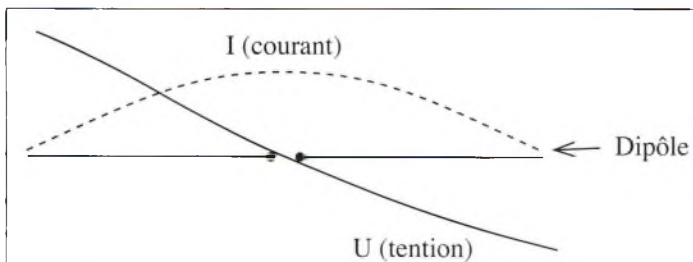
Fig. 2 — Au centre du doublet demi-onde, le courant est maximum et la tension nulle (ou au moins minimum).
