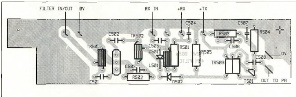
↑ ← Figure 5. Le filtre passe-bande HF (a) et l'implantation des composants (b).
