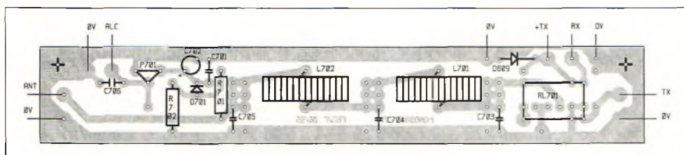
↑ ← Figure 7. Le filtre passe-bas (a) et l'implantation des composants (b).
