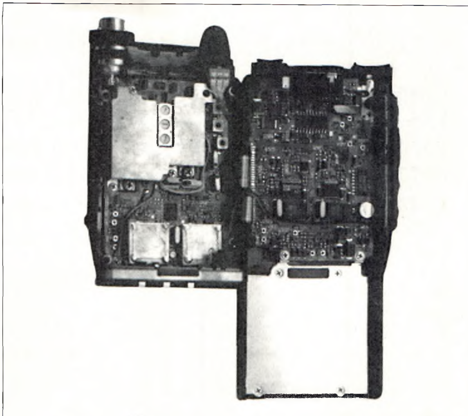
L'intérieur du DJ-G5E. Il y a deux circuits imprimés reliés à l'aide d'une nappe de fils (ruban). La présence de composants CMS est flagrante.
