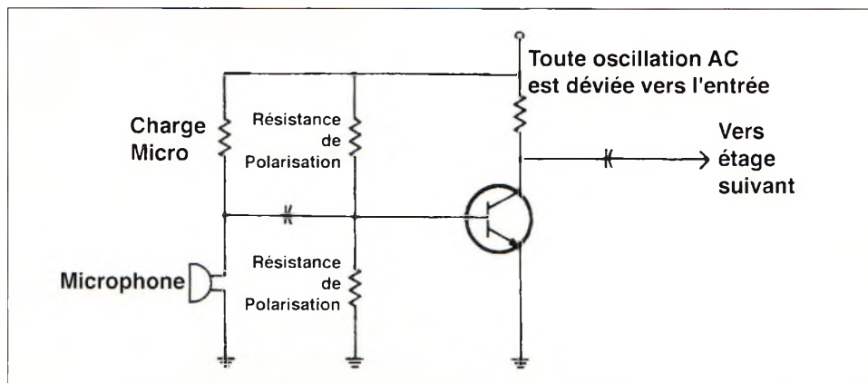
Figure 3. Etage d'entrée micro classique.
