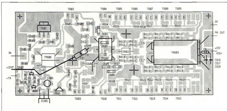
↑ ← Figure 6. Le bloc PA (a) et l'implantation des composants (b).
