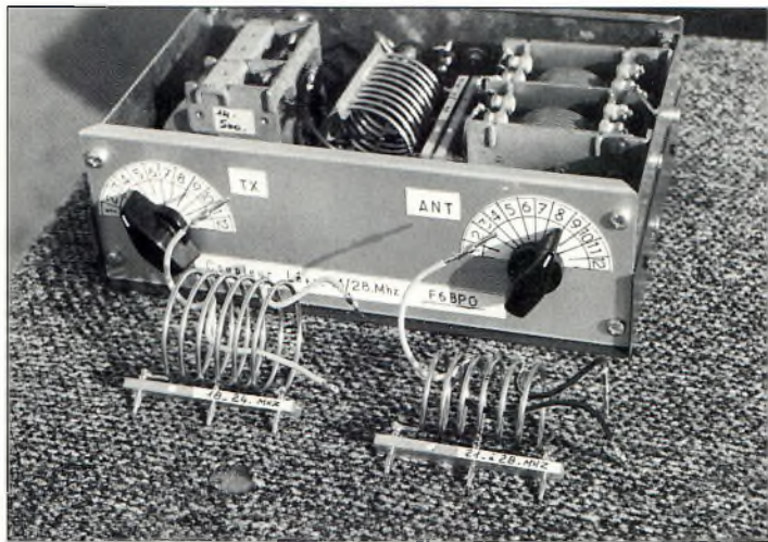
Photo 1. Boîte de couplage pour antenne Lévy type "Auto Transfo" à trois selfs interchangeables, s'enfichant horizontalement, permettant de couvrir la gamme 14-28 MHz. La puissance admissible est de 100 watts.
