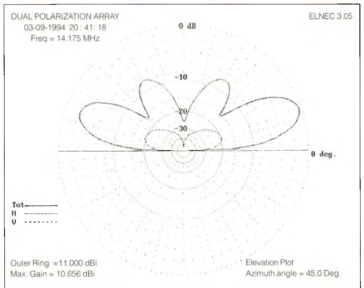
Figure 5. Diagramme de rayonnement calculé par ELNEC pour la bande 20 mètres d'après l'antenne décrite en figure 1, au-dessus d'un sol réel.
