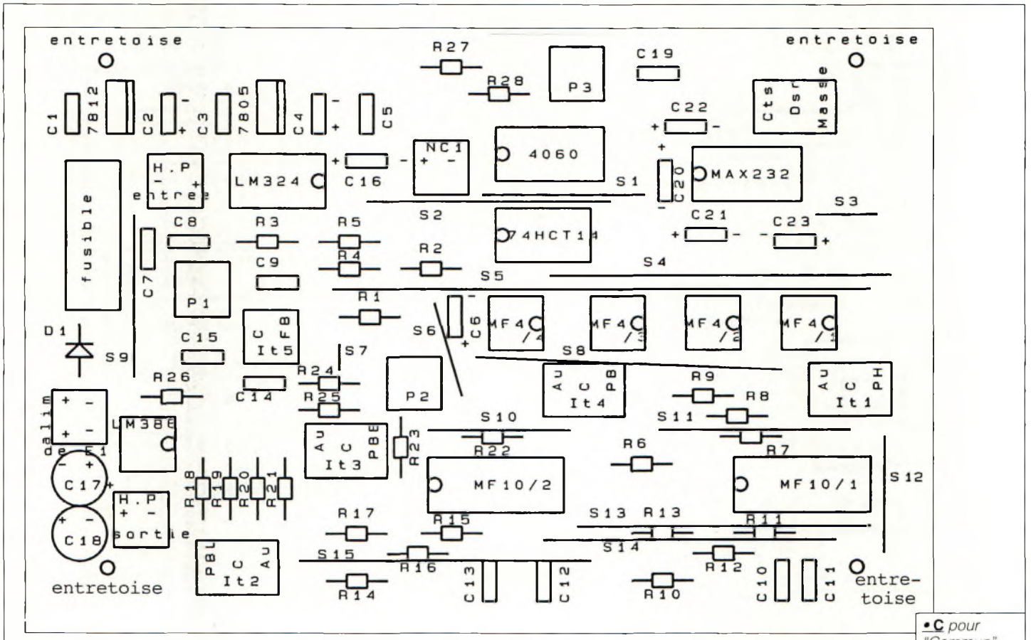
Figure 3. Le schéma de repérage.
