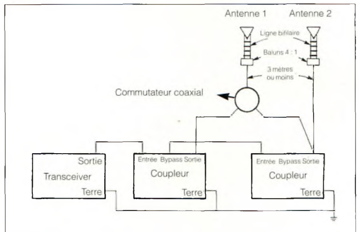
Figure 2. En utilisant le système décrit ici, on peut utiliser une seule antenne avec son coupleur indépendant, soit utiliser les deux antennes avec un coupleur unique. Les baluns peuvent être installés à l'extérieur du shack à condition que le coaxial fasse moins de 3 mètres de long.
