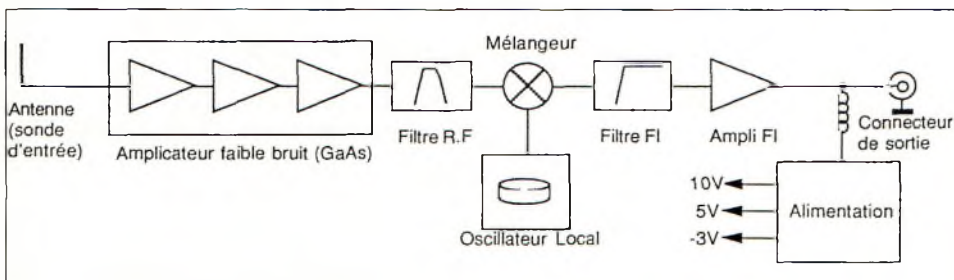
Synoptique d'un Low Noise Block (LNB)
