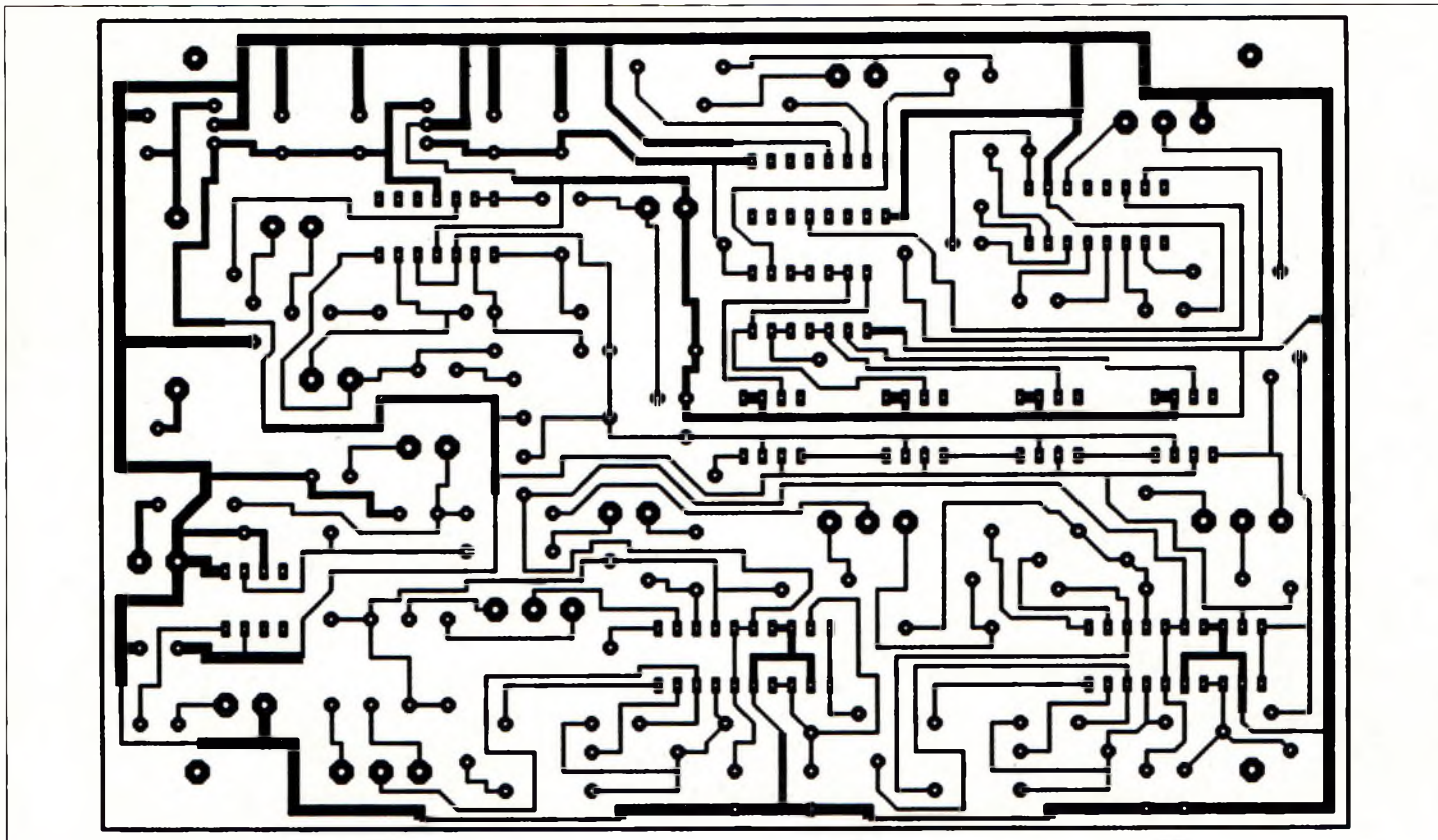
Figure 1. Le circuit Imprimé vu côté composants (Echelle 1:1).
