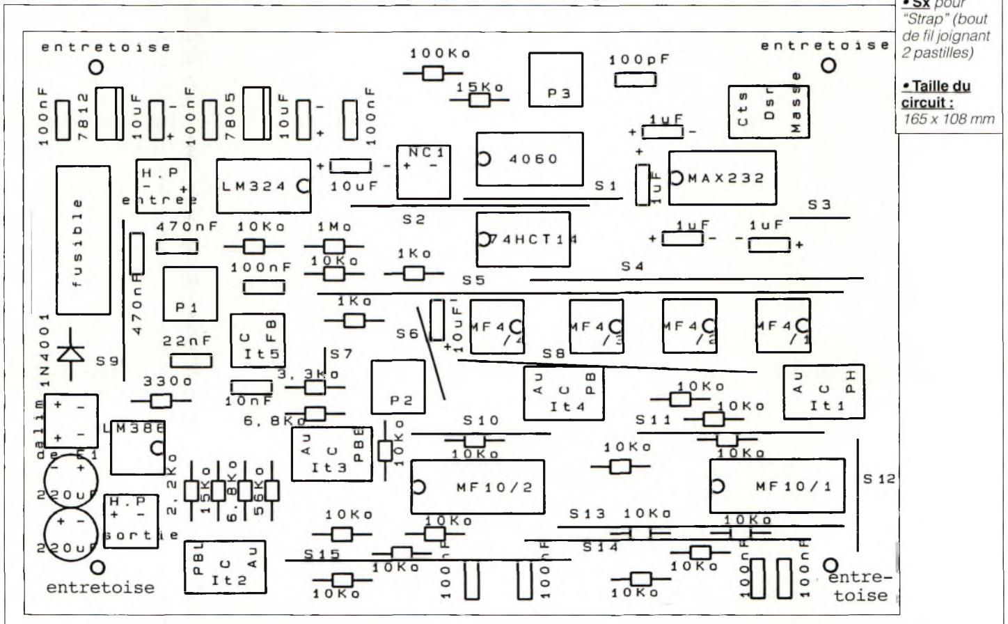
Figure 2. Le plan d'implantation des composants.
