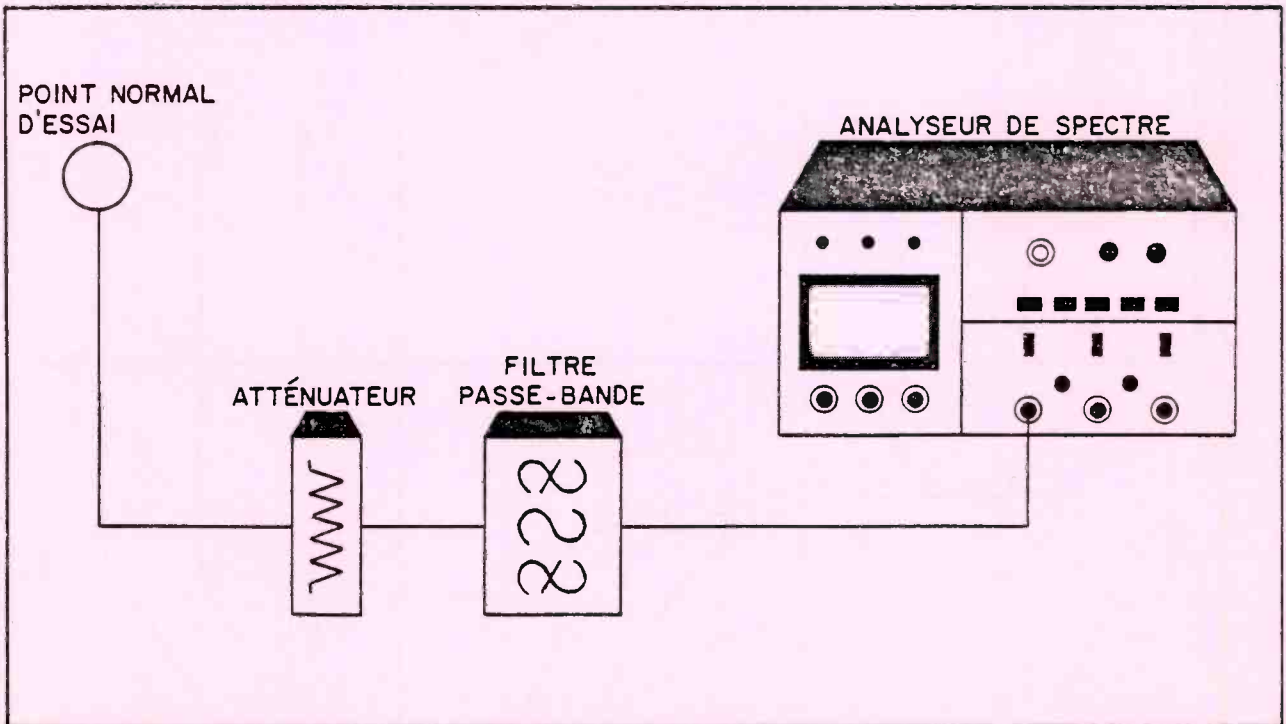
FIGURE 5-4 Montage du matériel d'essai pour la mesure du rapport porteuse/batttement et porteuse batttement composite.
