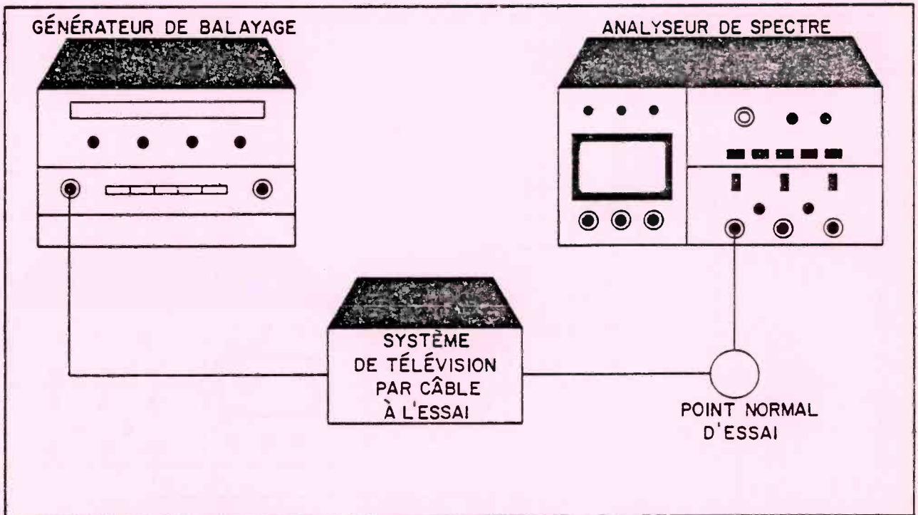
FIGURE 5-7 Montage du matériel d'essai pour la mesure de la réponse en fréquences du système à large bande.
