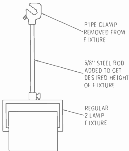
Fig. A-3. A light hanger.
