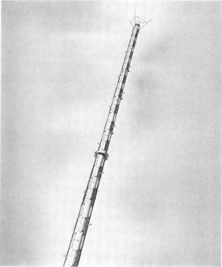
Fig. 7-1. The RCA slotted antenna. (RCA)
