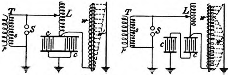
FIG. 115. SEIBT'S POTENTIAL INDICATOR. FIG. 116.
