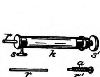
FIG. 66. THE BRAUN COHERER.
