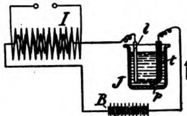
FIG. 113. WEHNELT INTERRUPTER.
