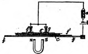
FIG. 47. MUIRHEAD FILINGS-COHERER.
