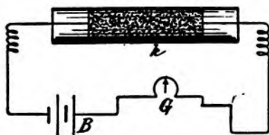
FIG. 10. BRANLY COHERER.
