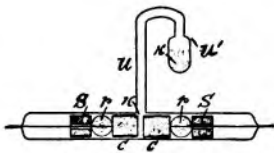
FIG. 74. BLONDEL COHERER.
