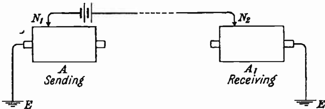
FIG. 10.—Bakewell's Apparatus.
