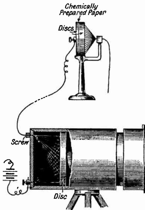
FIG. 15.—Carey's Apparatus,
