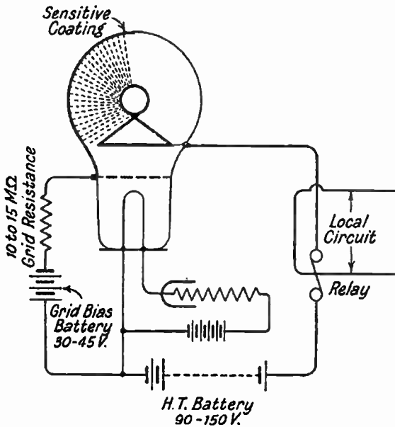
FIG. 50.—Zworykin's Cell.
