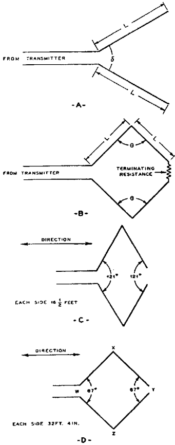
Fig. 64 Diamond and "V" Antennas.
