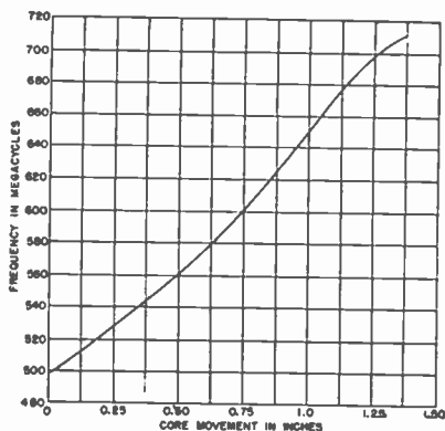
Fig. 11—Tuning curve.
