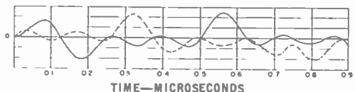
(d) Voltage on the red kinescope grid.
