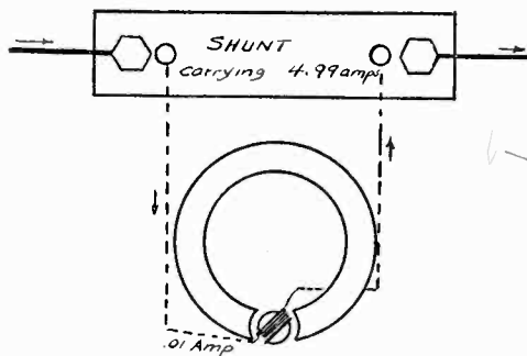
Fig. 4. Ammeter Shunt.
