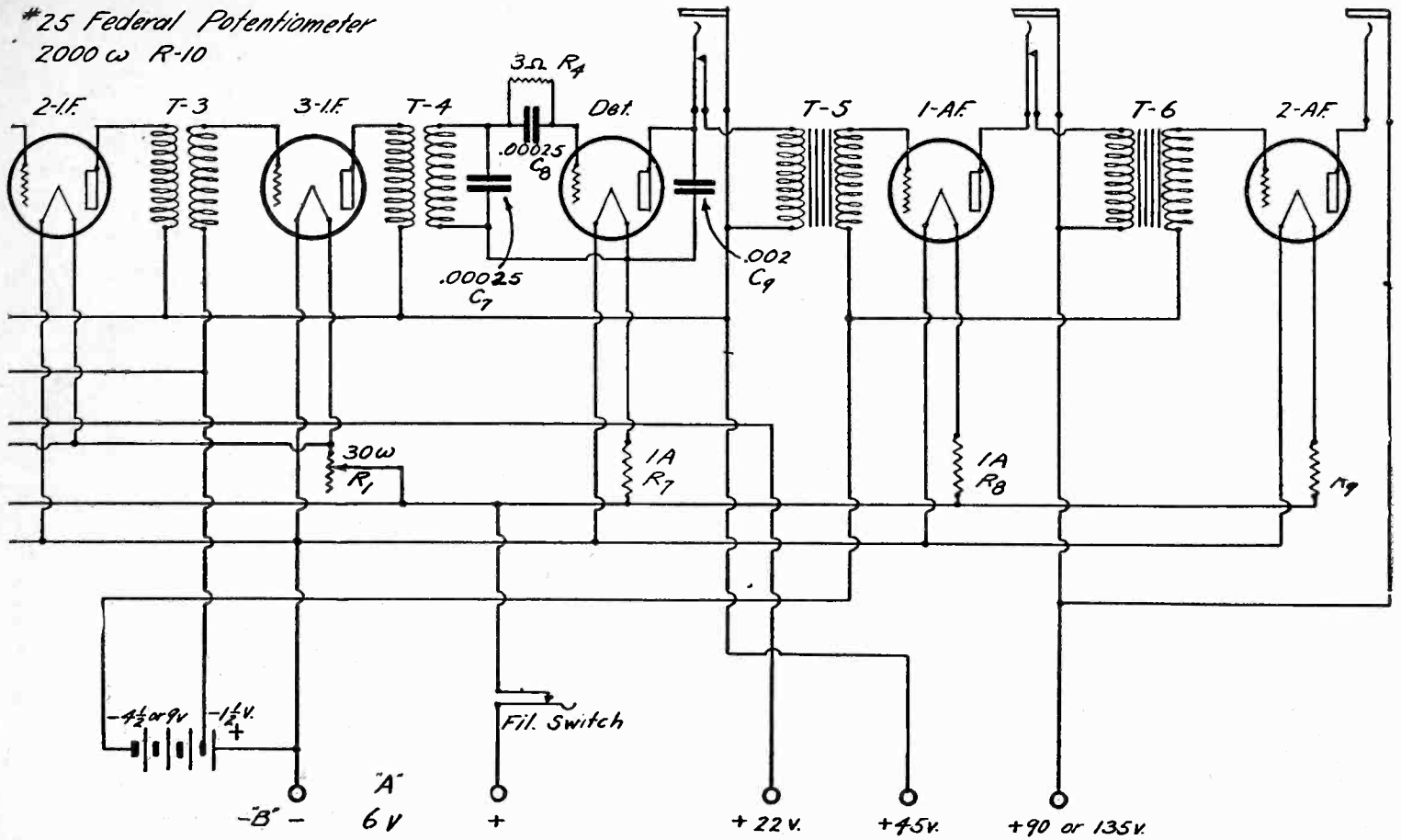
Fig. 3. Schematic Wiring Diagram.
