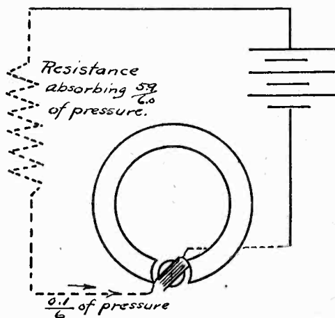
Fig. 5. Voltmeter Shunt.
