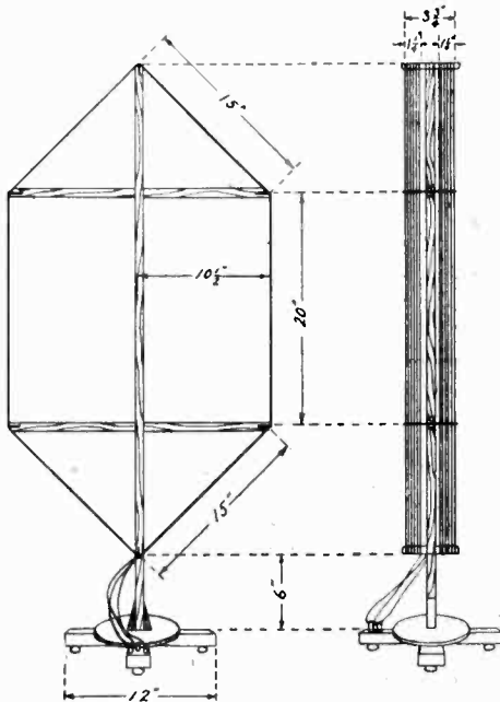
Fig. 7. Center Tap Loop Antenna.
