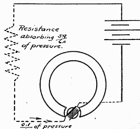
Fig. 5. Voltmeter Shunt.
