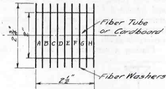
Fig. 1. Core Dimensions
