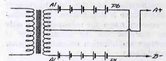
Rectifier Assembly
