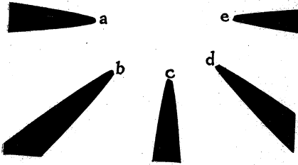
Fig. 8. Needle wear. a. unused b. 5 min. c. 10 min. d. 15 min. e. 20 min.
