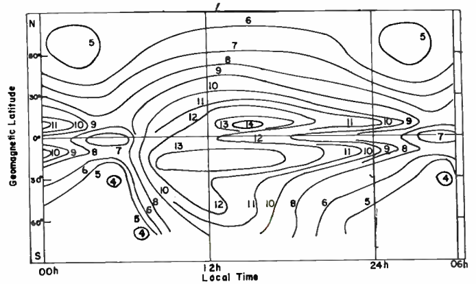
Fig. 4— f_0F_2 1947. N. Solstice.
