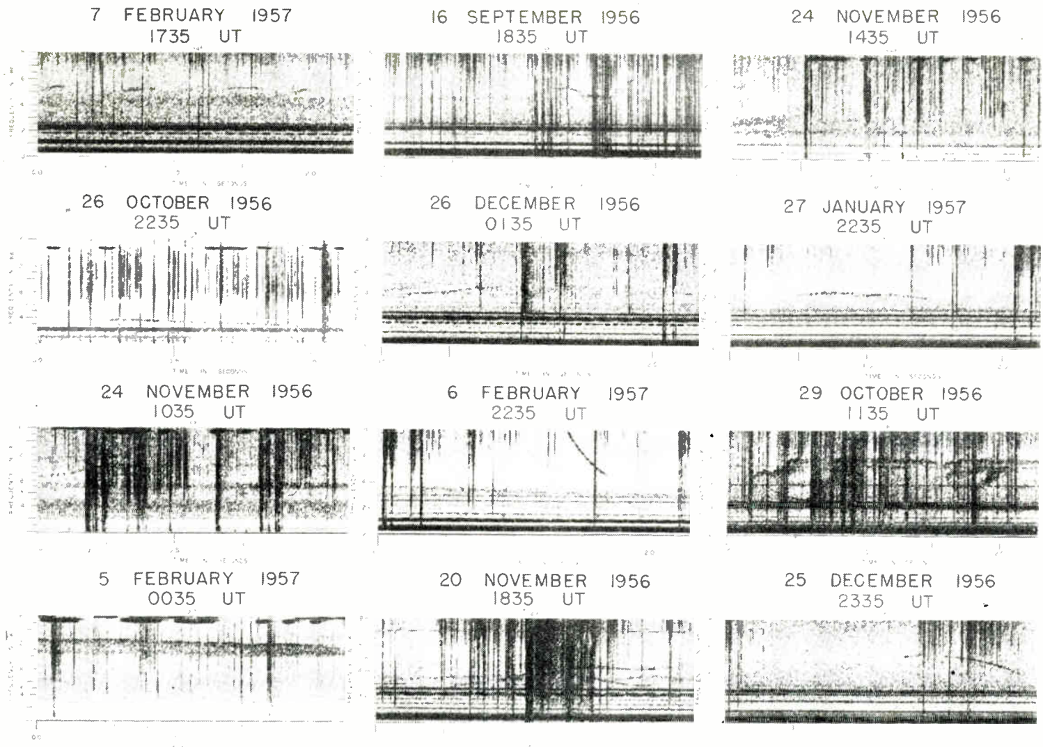
Fig. 8—Quasi-horizontal tones.
