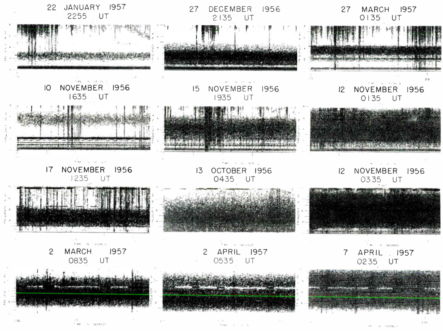
Fig. 11—Hiss.
