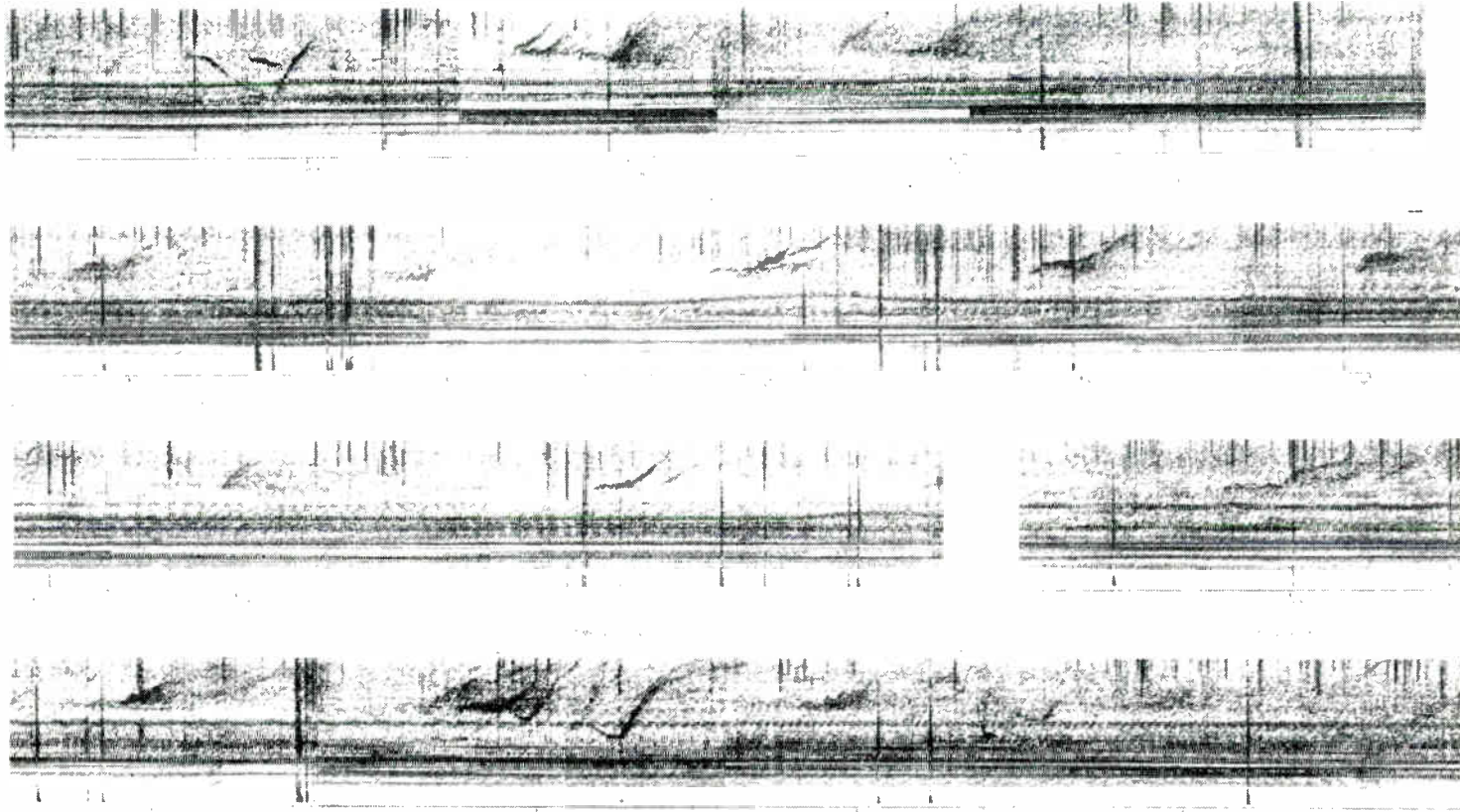
Fig. 6—Alaska.
