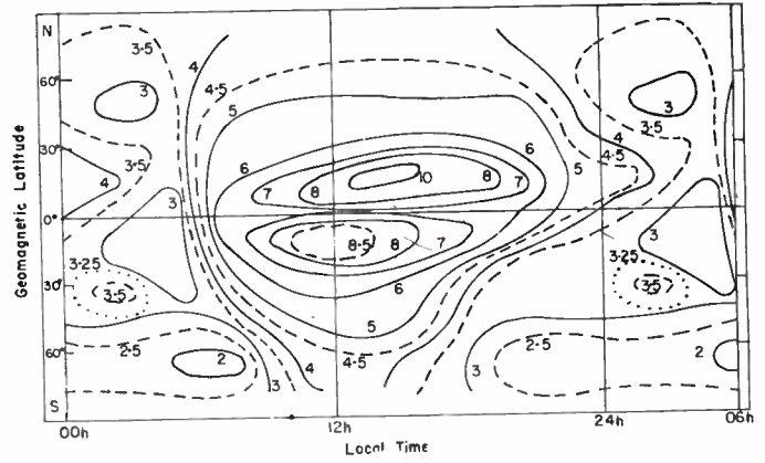
Fig. 3— f_0F_2 1943-1944. N. Solstice.
