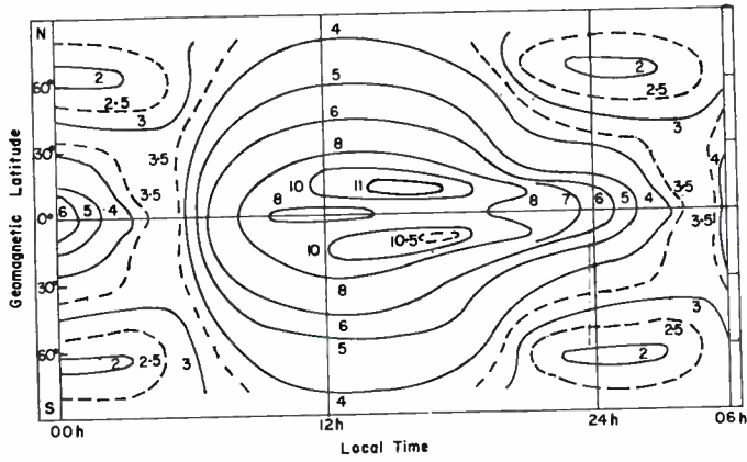
Fig. 1— f_0F_2 1943-1944. Equinox.
