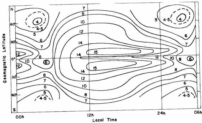
Fig. 2— f_0F_2 1947. Equinox.
