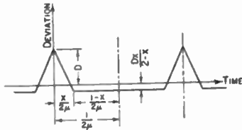
Fig. 14—Modulating signal.
