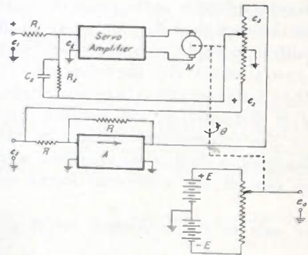
Fig. 11—Servodivider circuit.
