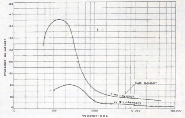
(d) Inductance of a VR75 tube.
