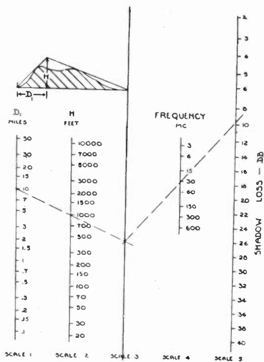
Fig. 4—Shadow loss.
