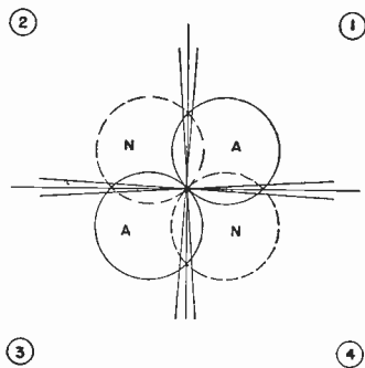
Fig. 1—Four-course radio range.
