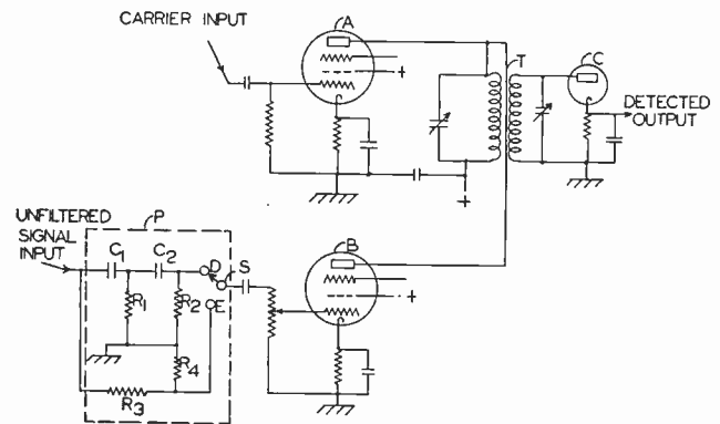
Fig. 5—Single-diode detector circuit.
