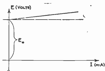
Fig. 1—Gas-tube characteristic.
