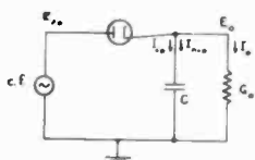
Fig. 1—Simple diode rectifier circuit.
