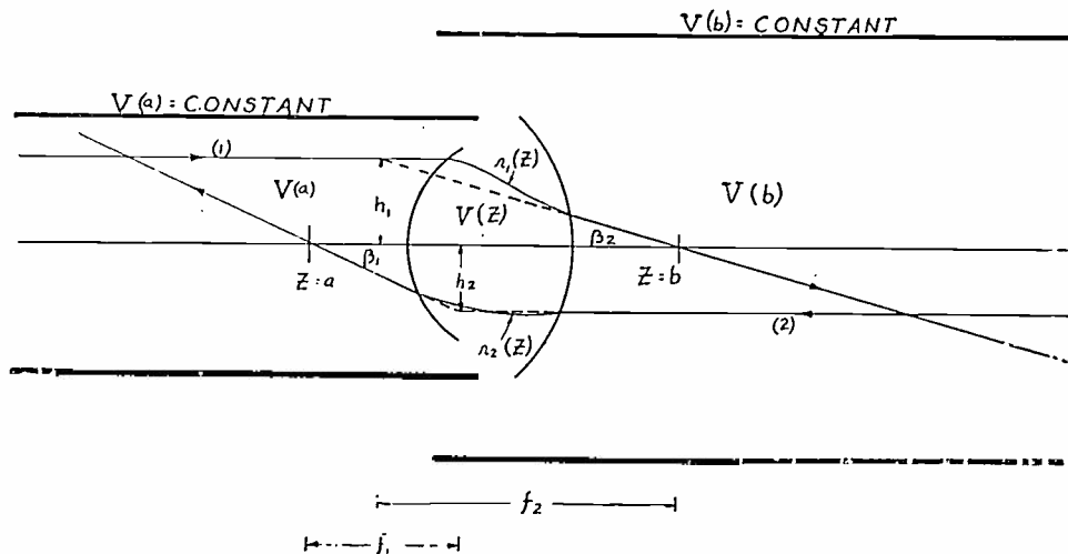
Fig. 4—Two fundamental trajectories.
