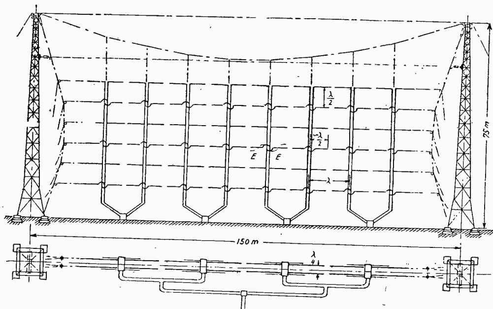
Fig. 8—Telefunken aerial.
