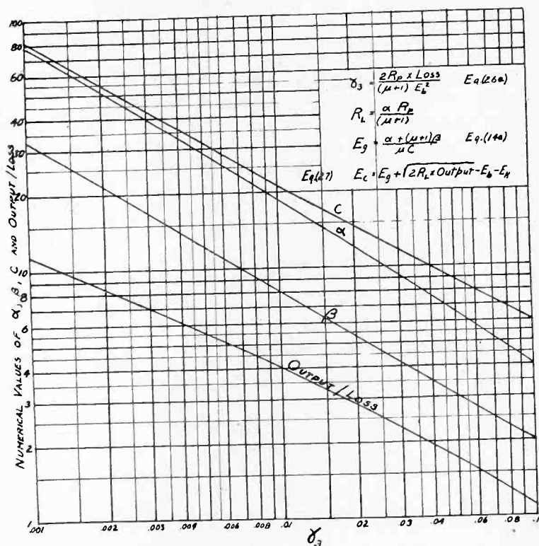
Fig. 12—Design data.
