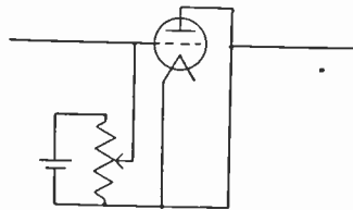
Fig. 6—Electronic oscillator circuit, Barkhausen-Kurz, 1920.
