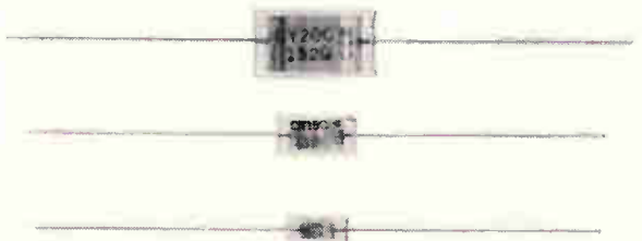
CORNING CYFM Capacitors: CYFM 10, 0.5—300 pf; CYFM 15, 220—1200 pf; CYFM 20, 560—5100 pf; CYFM 30, 3600—10,000 pf; VDCW, 300 and 500 volts.
