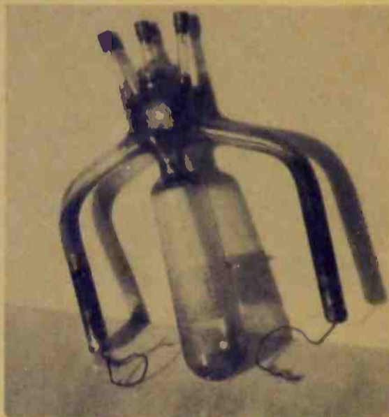
Fig. 3 A Cooper Hewitt mercury-arc rectifier tube.
