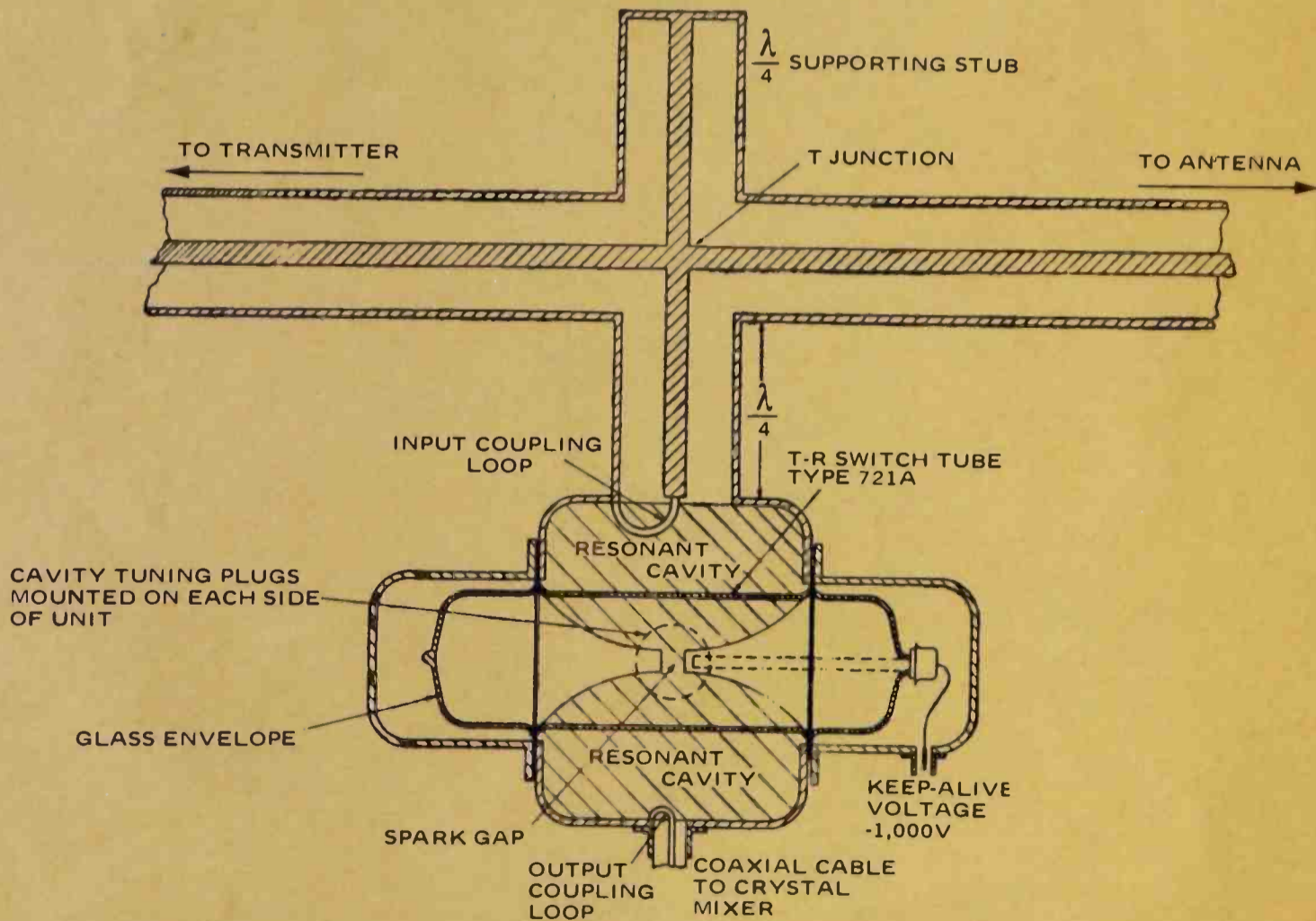
Fig. 25 A T-R tube arrangement.
