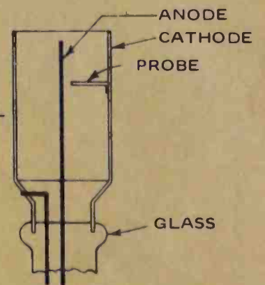
Fig. 22 A strobotron tube.
