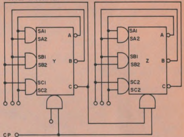
MODULE 9 COUNTER
