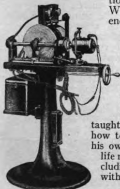
One of the Electrical Test Tables used at M. S. A. S.
