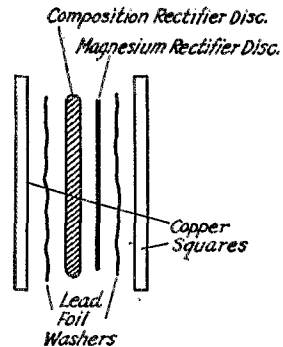
FIG. 1—A SINGLE RECTIFIER ASSEMBLY
