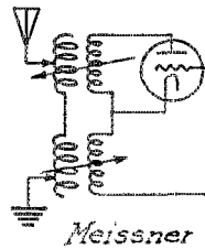
Meissner
