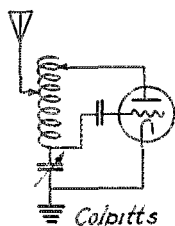
Colpitts
