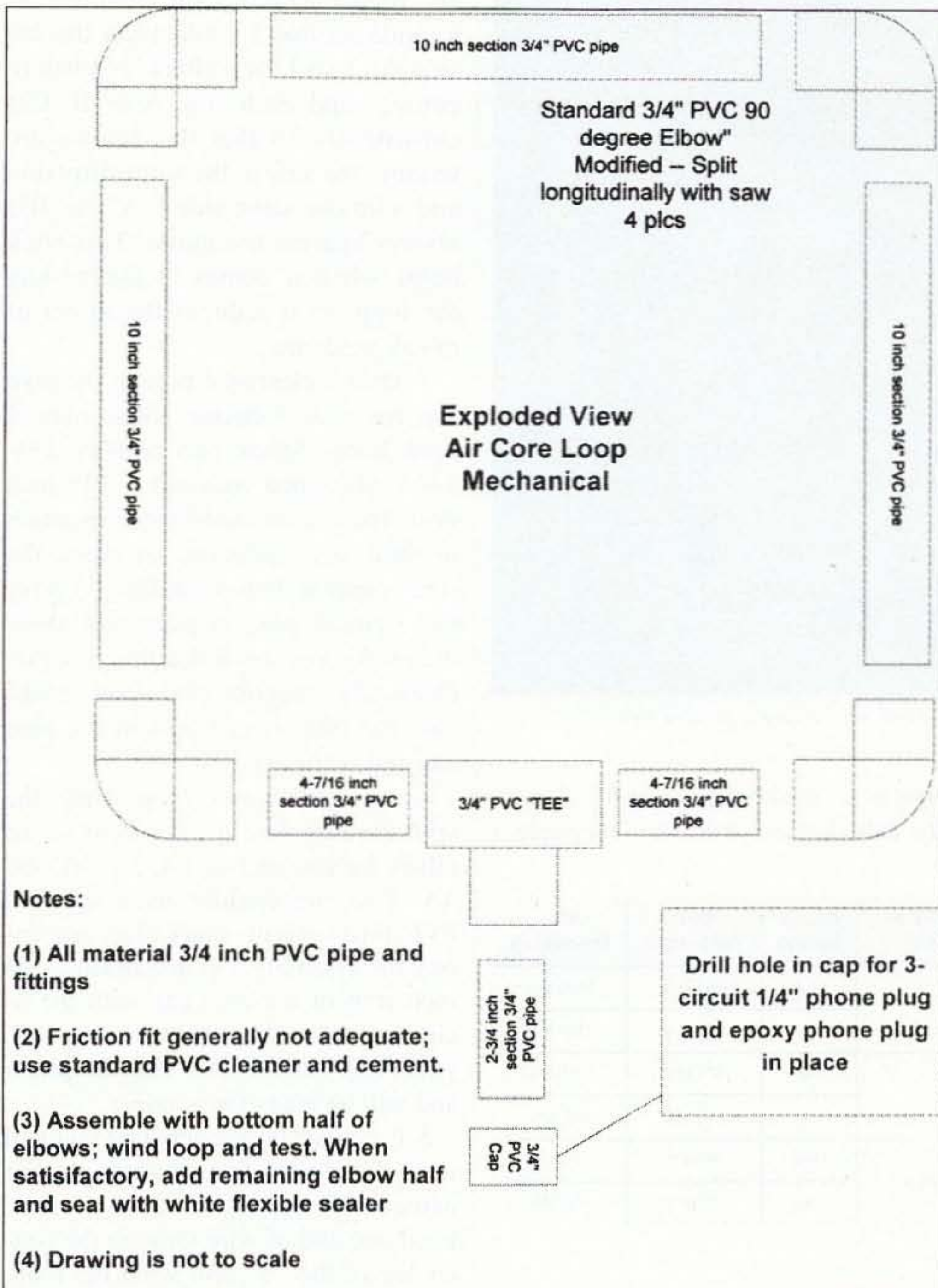
Fig. 8. Air core loop.
