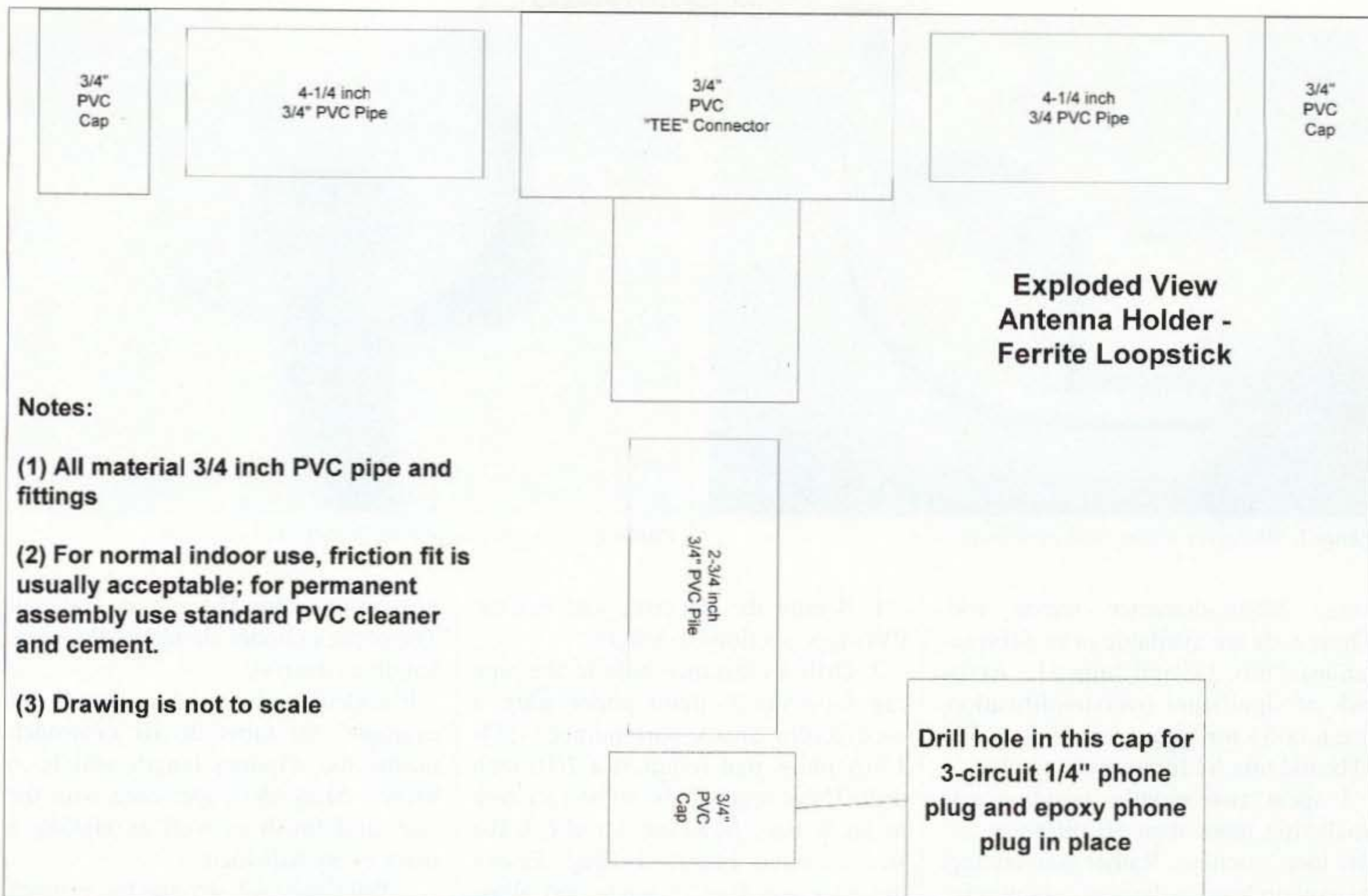
Fig. 9. Ferrite loop.
