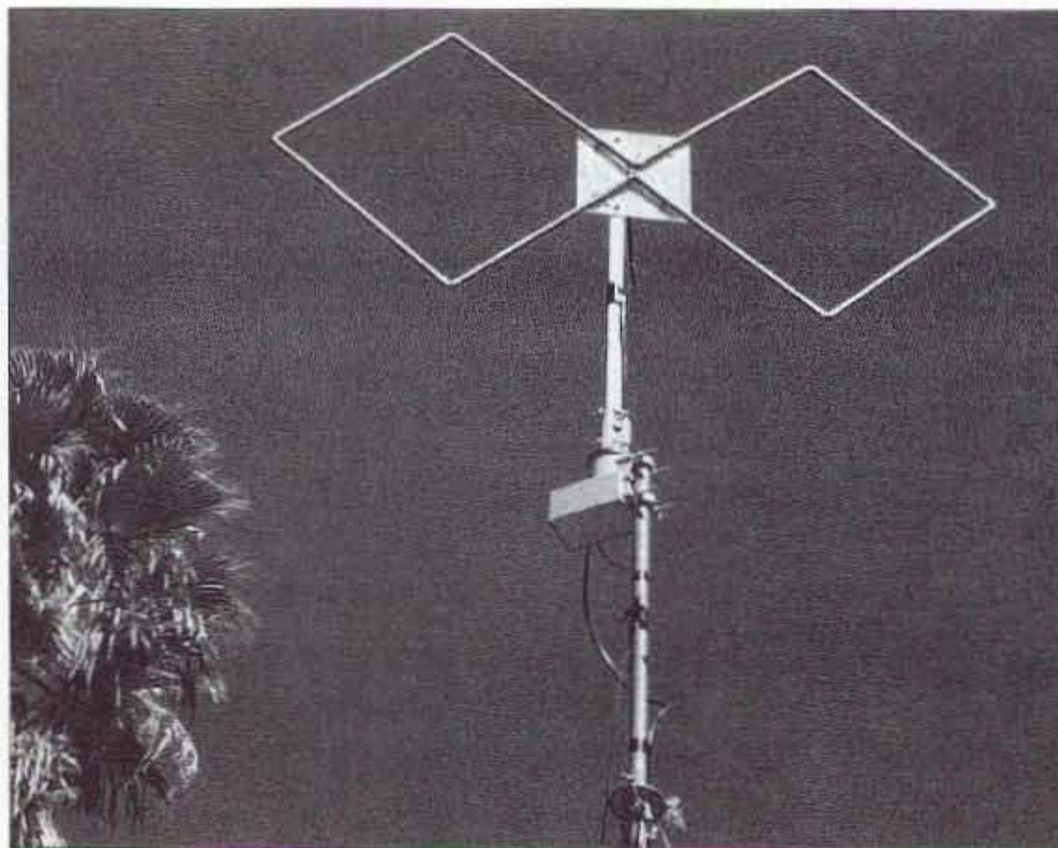
Photo A. 2m twin loop antenna.
