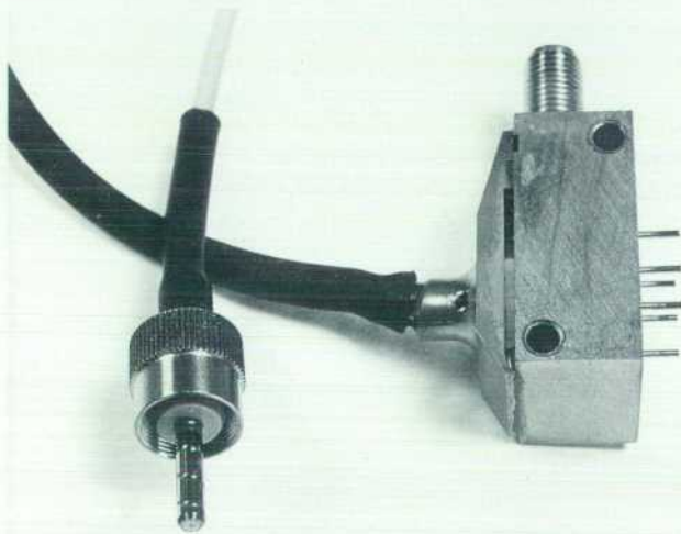
Fig. 10. HP 83481A O/E converter.
