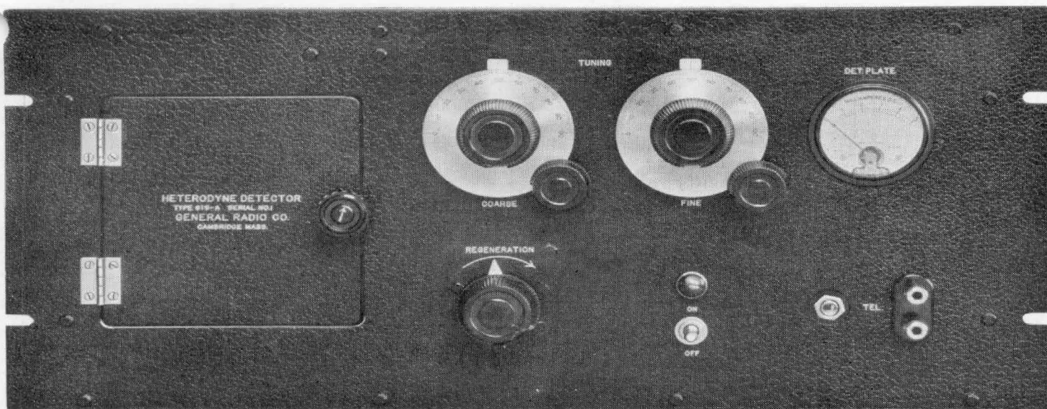
TYPE 619-A Heterodyne Detector
