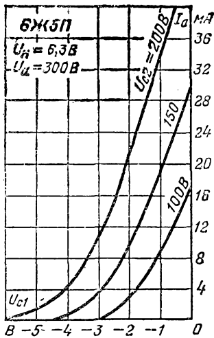
Анодно-сеточные характеристики.
