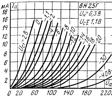
Анодные характеристики.
