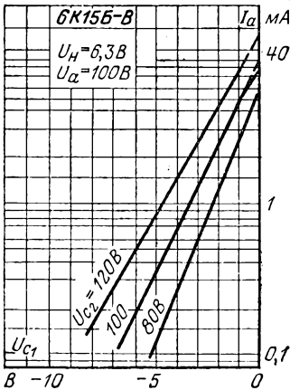
Анодно-сеточные характеристики.
