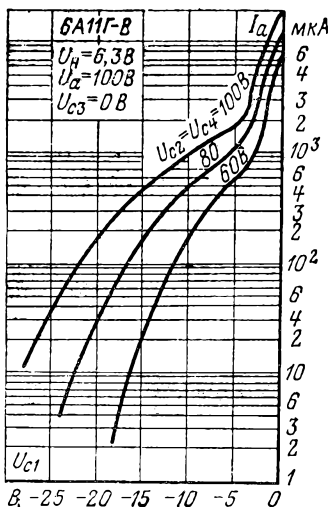
Анодно-сеточные характеристики.
