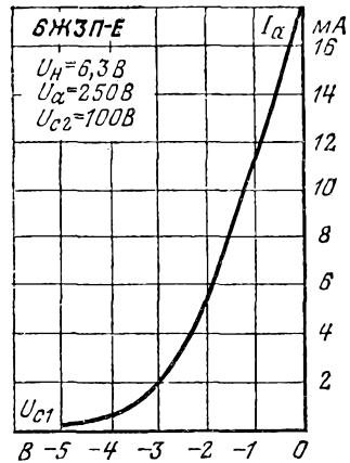
Анодно-сеточная характеристика.
