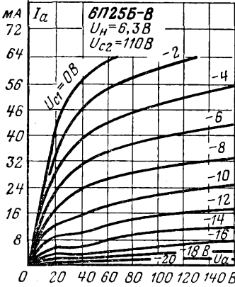
Анодные характеристики.
