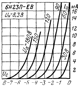
Анодно-сеточные характеристики.
