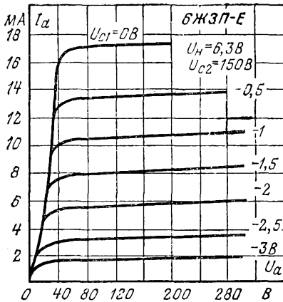
Анодные характеристики.
