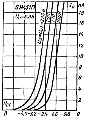
Анодно-сеточные характеристики.
