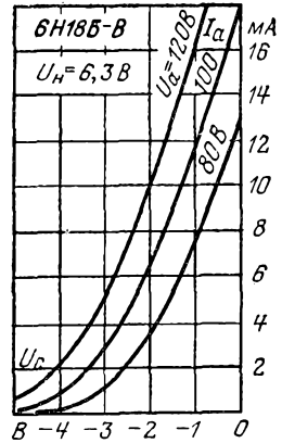
Анодно-сеточные характеристики.
