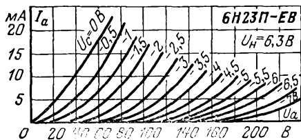
Анодные характеристики.
