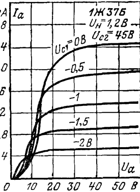
Анодные характеристики.
