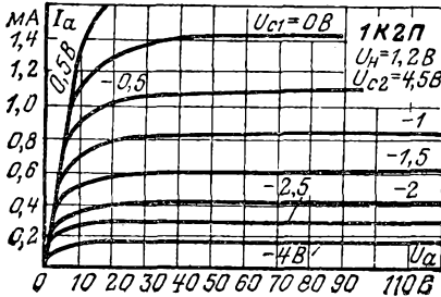
Анодные характеристики.
