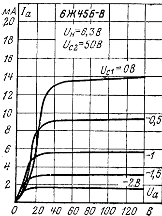
Анодные характеристики.
