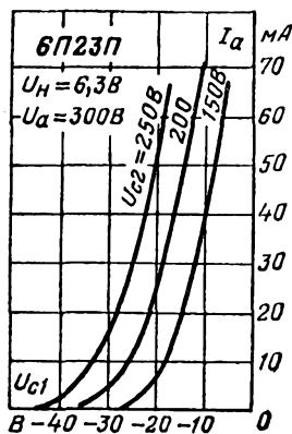
Анодно-сеточные характеристики.
