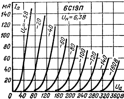
Анодные характеристики,
