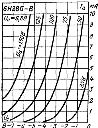
Анодно-сеточные характеристики
