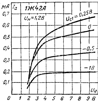
Анодные характеристики.
