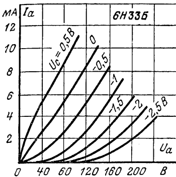
Анодные характеристики.
