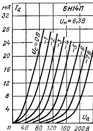
Анодные характеристики.
