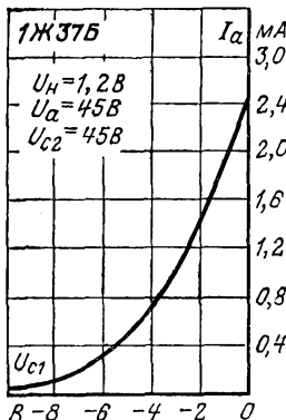
Анодно-сеточная характеристика по 1-й сетке (сетки C'_1 и C''_1 соединены).
