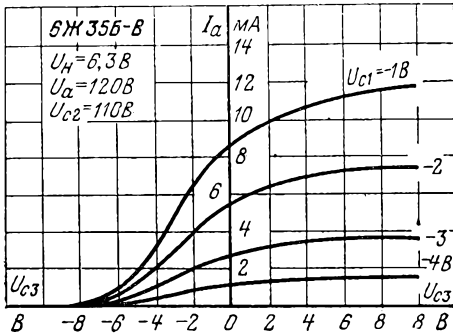
Анодно-сеточные характеристики по 3-й сетке.
