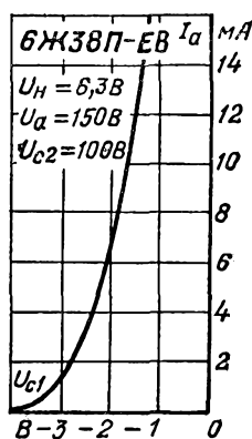
Анодно-сеточная характеристика.
