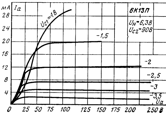
Анодные характеристики.
