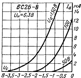
Анодно-сеточные характеристики.
