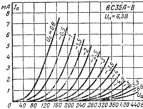
Анодные характеристики.
