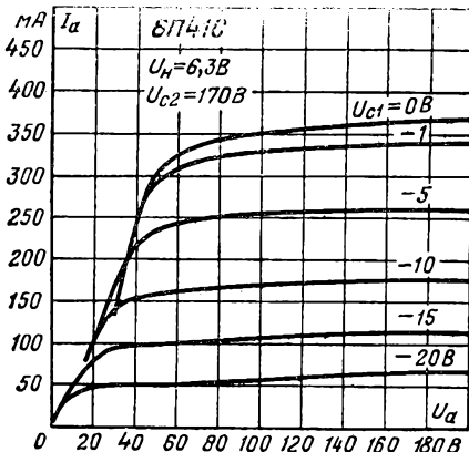
Анодные характеристики.
