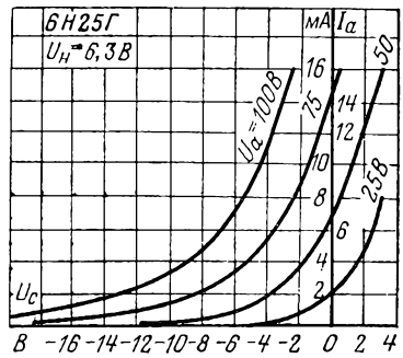
Анодно-сеточные характеристики.
