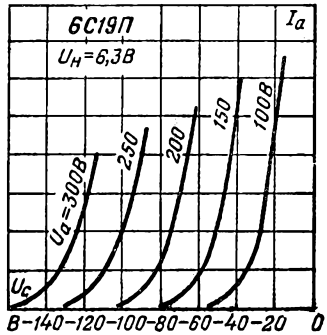
Анодно-сеточные характеристики.
