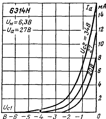
Анодно-сеточные характеристики.
