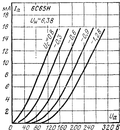
Анодные характеристики.
