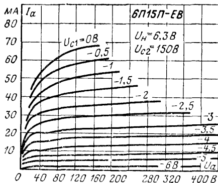
Анодные характеристики.
