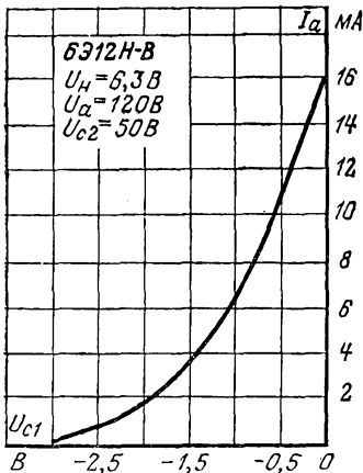
Анодно-сеточные характеристики.
