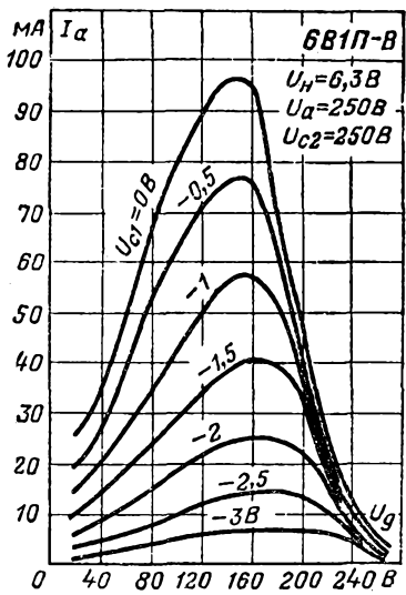
Анодно-катодные характеристики.
