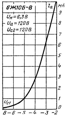
Анодно-сеточная характеристика.
