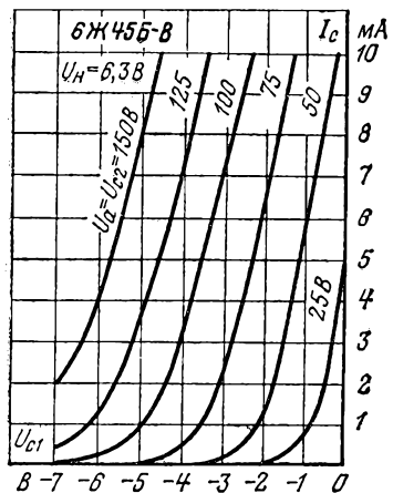
Анодно-сеточные характеристики.
