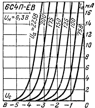
Анодно-сеточные характеристики.
