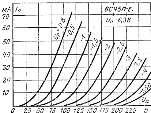
Анодные характеристики.
