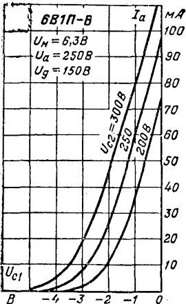
Анодно-сеточные характеристики.
