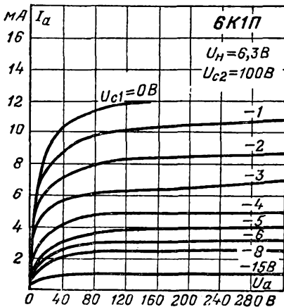
Анодные характеристики.
