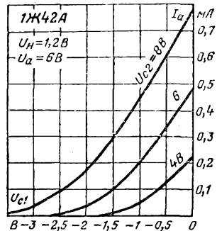
Анодно-сеточные характеристики по 1-й сетке.
