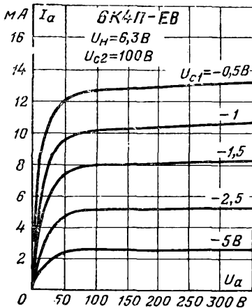
Анодные характеристики.
