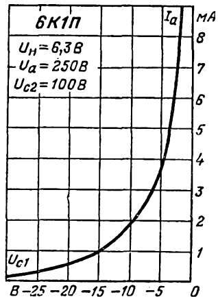
Анодно-сеточная характеристика.
