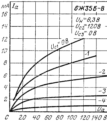
Анодные характеристики.
