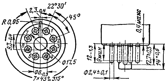
Присоединительные размеры ламп с октальным цоколем.
