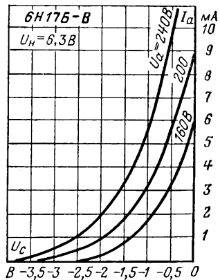
Анодно-сеточные характеристики.
