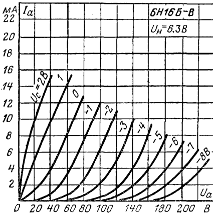
Анодные характеристики.
