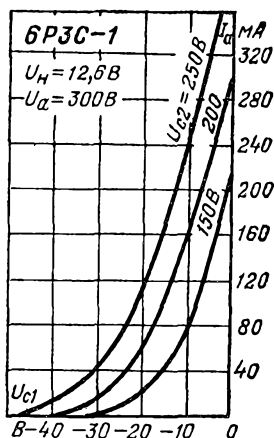
Анодно-сеточные характеристики.
