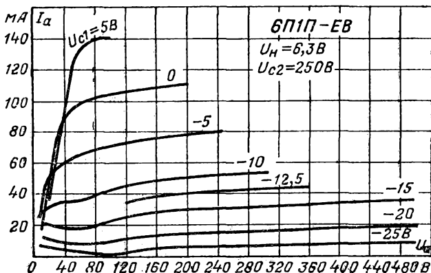
Анодные характеристики.
