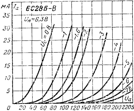
Анодные характеристики.
