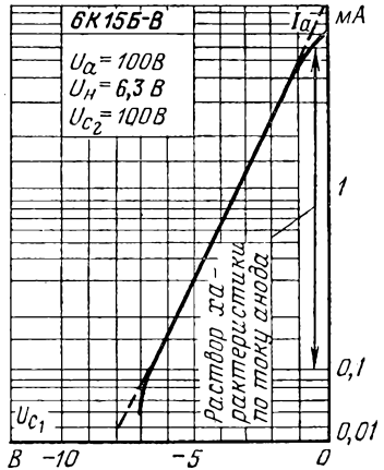
Анодно-сеточная характеристика.
