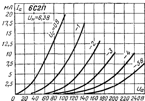
Анодные характеристики.
