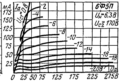
Анодные характеристики пентодной части.
