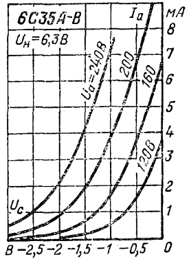
Анодно-сеточные характеристики.
