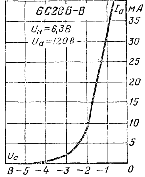
Анодно-сеточные характеристики.
