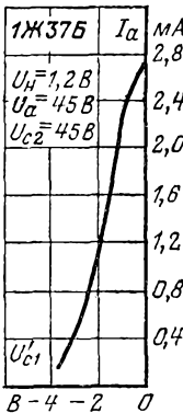
Анодно-сеточная характеристика по сетке C'_1 .
