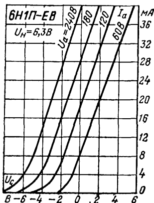
Анодно-сеточные характеристики.
