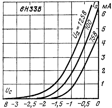
Анодно-сеточные характеристики.
