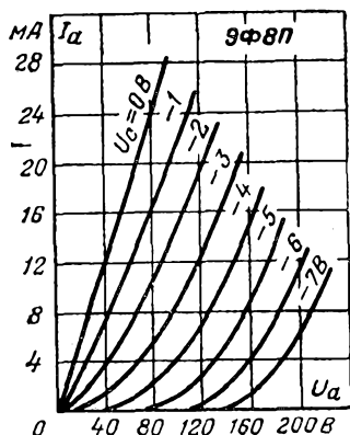
Анодные характеристики триодной части.
