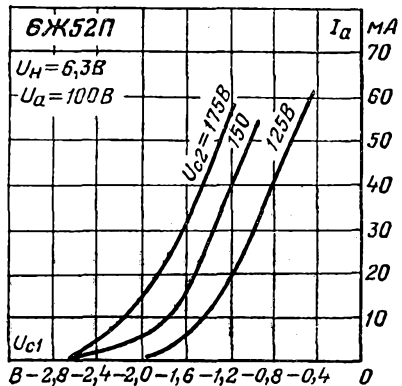
Анодно-сеточные характеристики.
