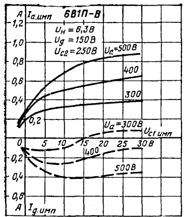
Импульсные анодно-сеточные (сплошные) и катодно-сеточные (пунктирные) характеристики.
