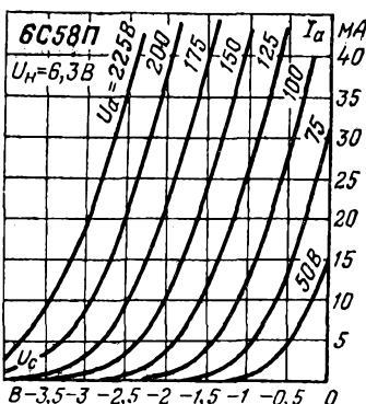
Анодно-сеточные характеристики.
