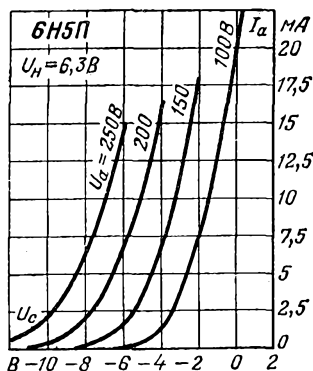
Анодно-сеточные характеристики.
