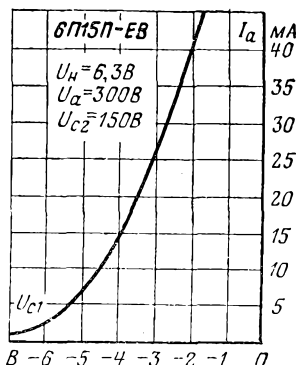
Анодно-сеточная характеристика.
