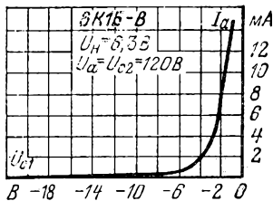
Анодно-сеточные характеристики.
