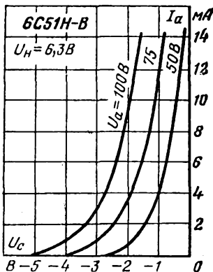
Анодно-сеточные характеристики.
