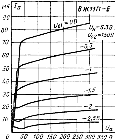
Анодные характеристики.
