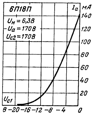
Анодно-сеточная характеристика.
