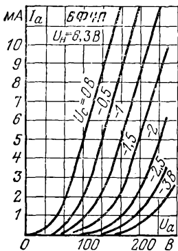
Анодные характеристики триодной части.
