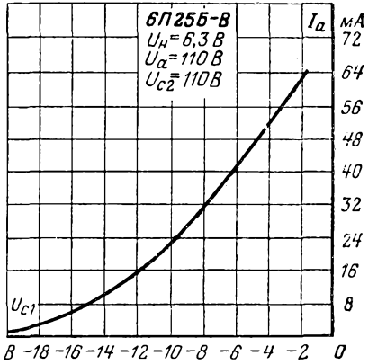
Анодно-сеточная характеристика.
