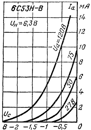
Анодно-сеточные характеристики.
