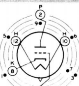
INDEX - LARGE LUG • - SHORT PIN - IC
