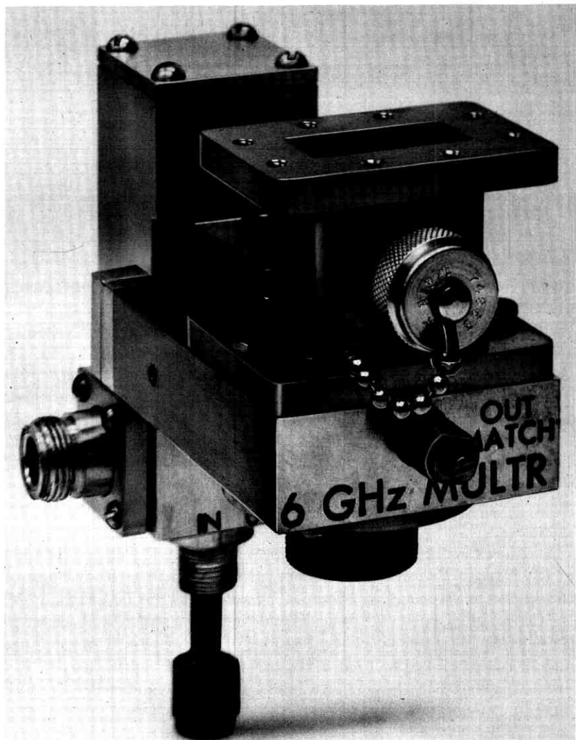
Fig. 11—Sextupler.
