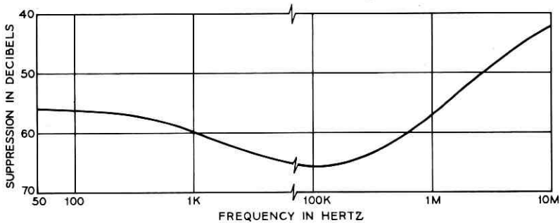
Fig. 17—4A FM terminal pair: longitudinal suppression.
