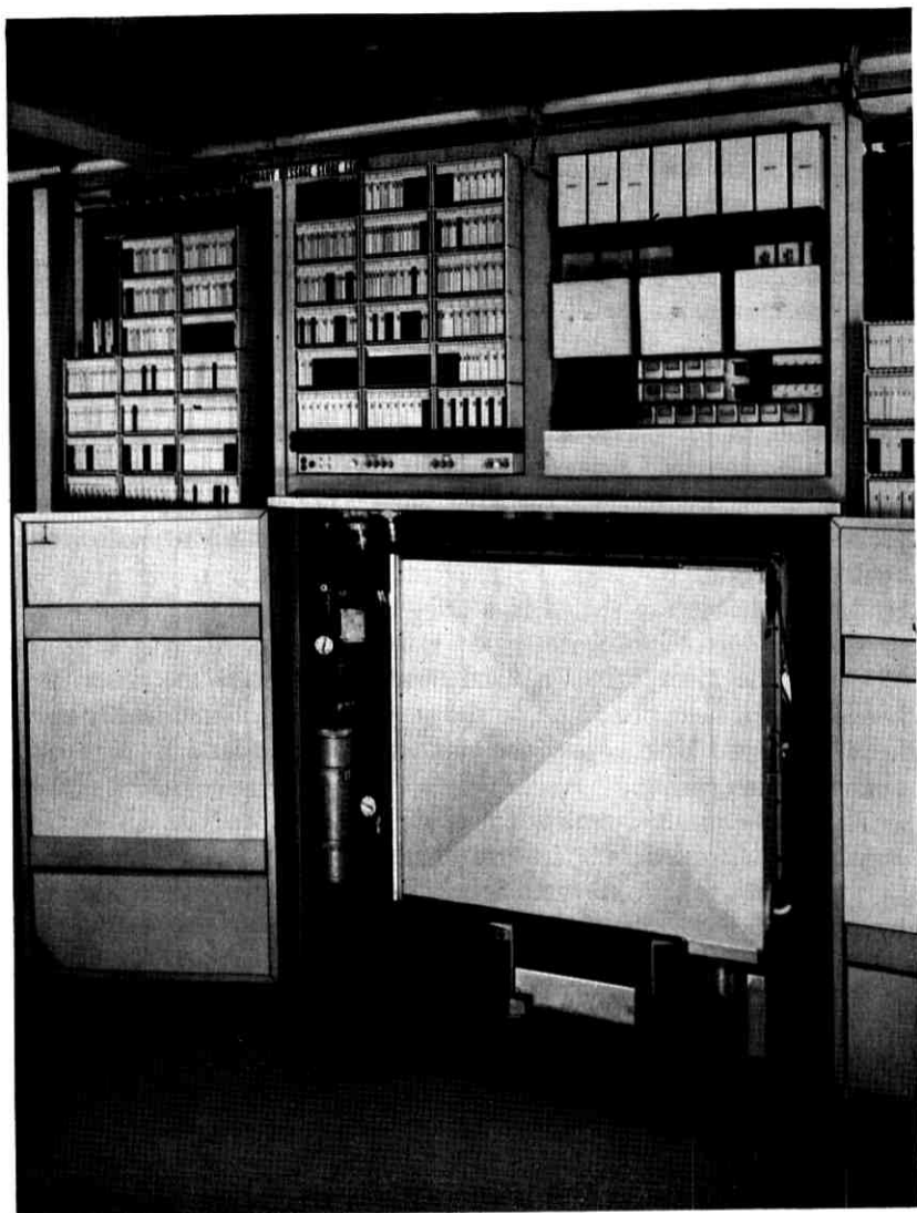
Fig. 2—Message store.
