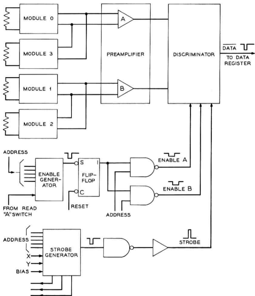
Fig. 15—Readout system.
