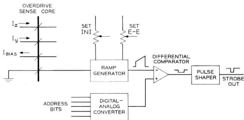
Fig. 18—Strobe generator.
