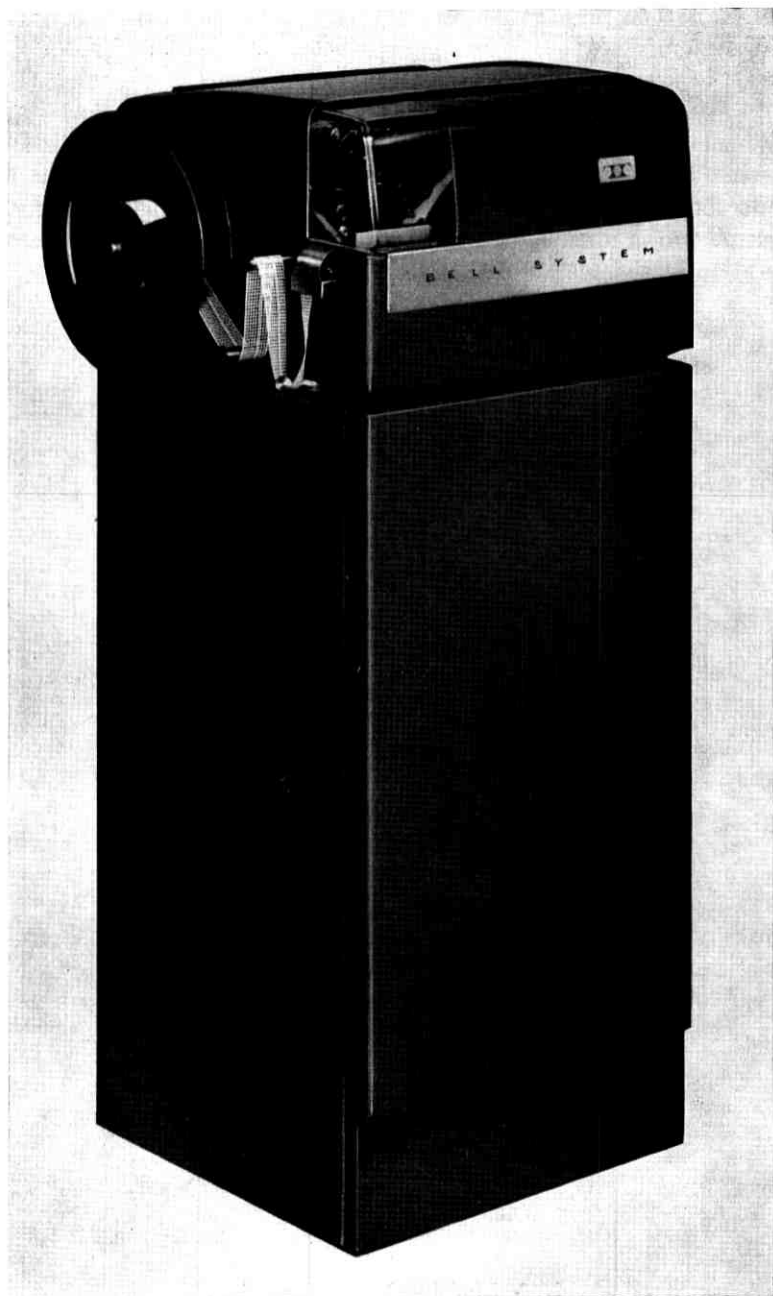
Fig. 10—Model 37 ROTR.
