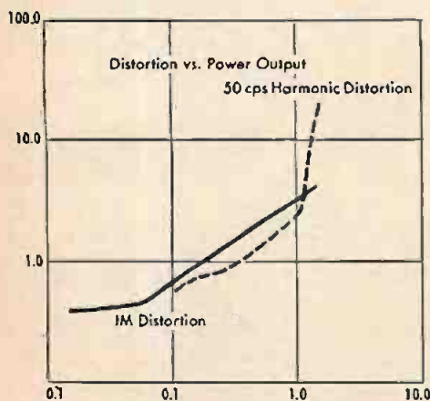
Harmonic and IM distortion.
