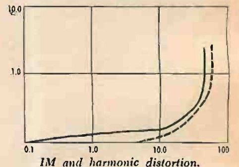
IM and harmonic distortion.
