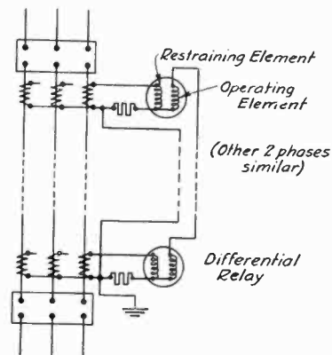
FIG. 2—PILOT WIRES
