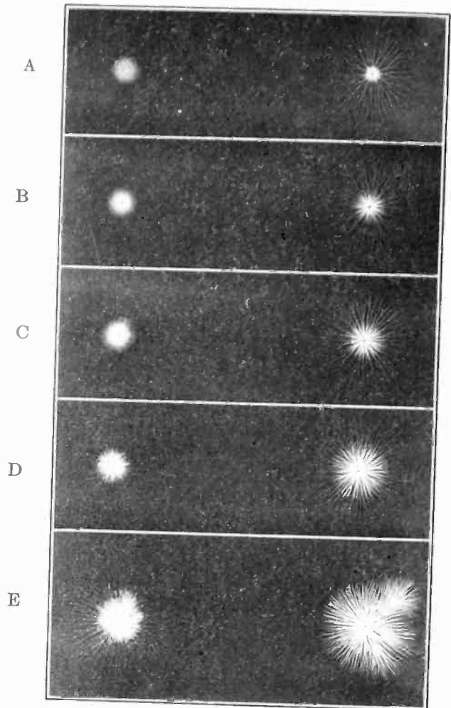
FIG. 1—LICHTENBERG FIGURES
