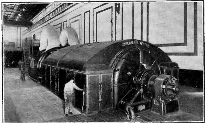
FIG. 2—160,000-Kw. GENERATOR
