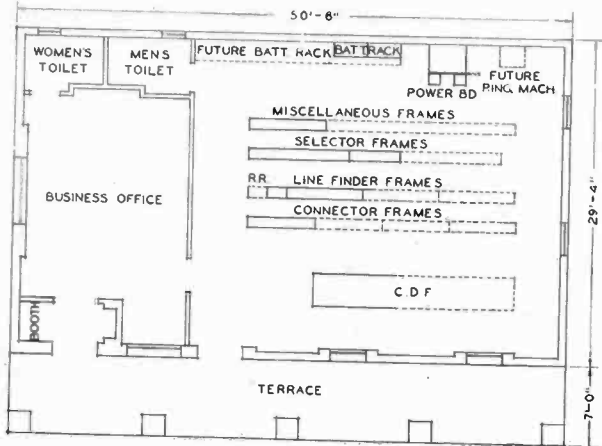
FIG. 6—FLOOR PLAN, OJAI
