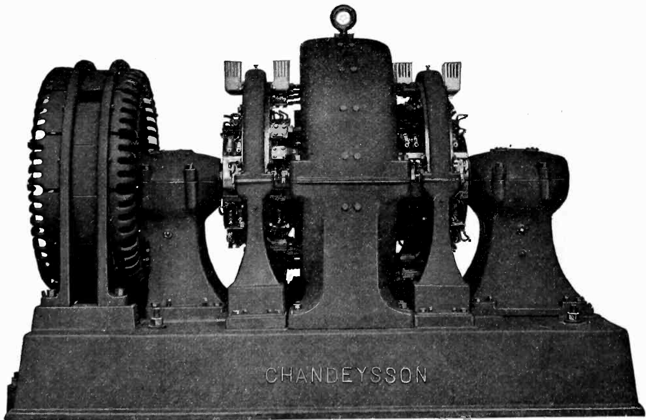
5000-amp., 6-volt; 2500-amp., 12-volt Generator
